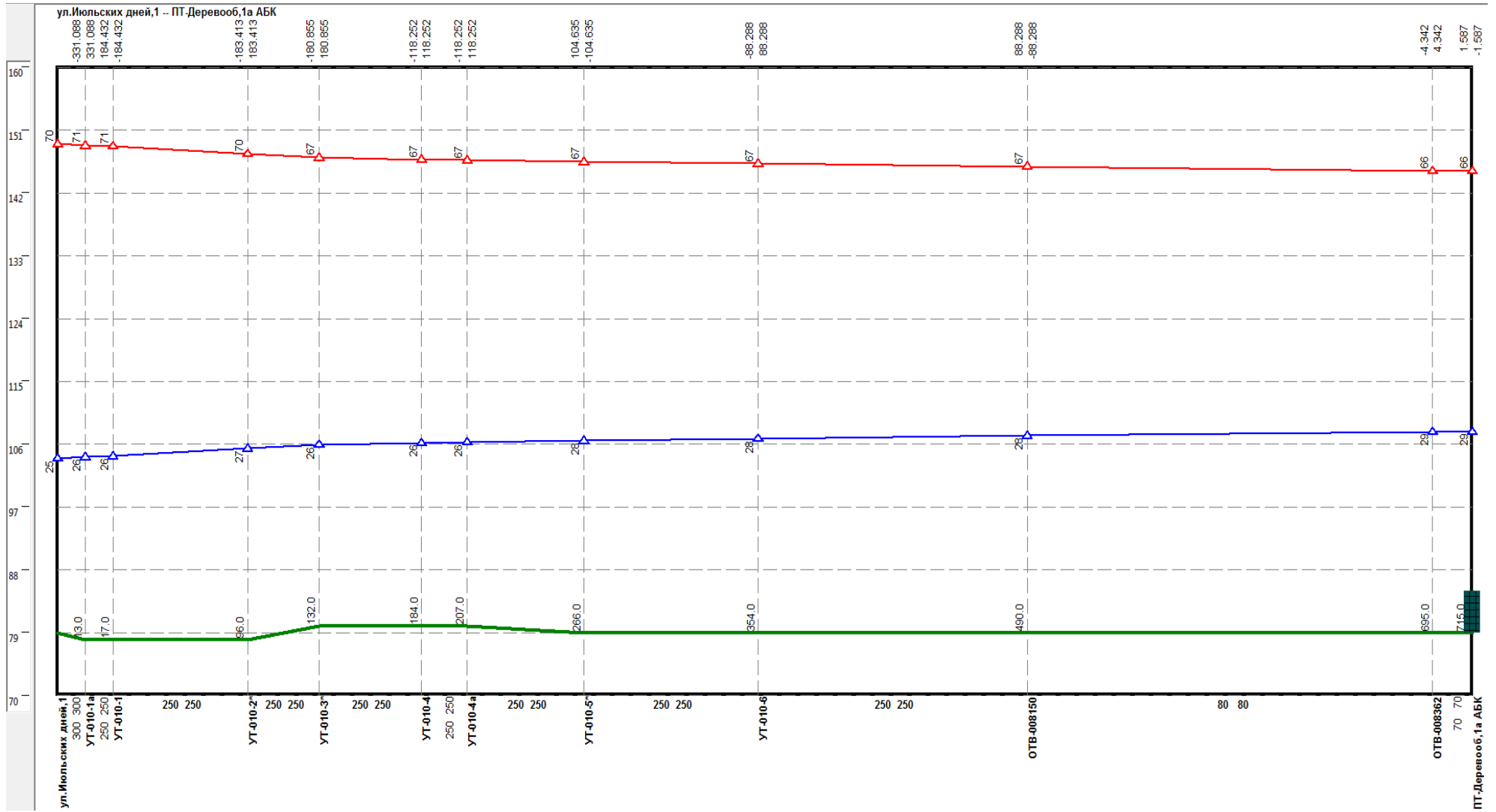
Рисунок 0.34 –Результат гидравлического расчета - график гидравлических режимов по пути теплоносителя от Июльских дней, 1 до ПТ-Деревооб, 1а АБК
