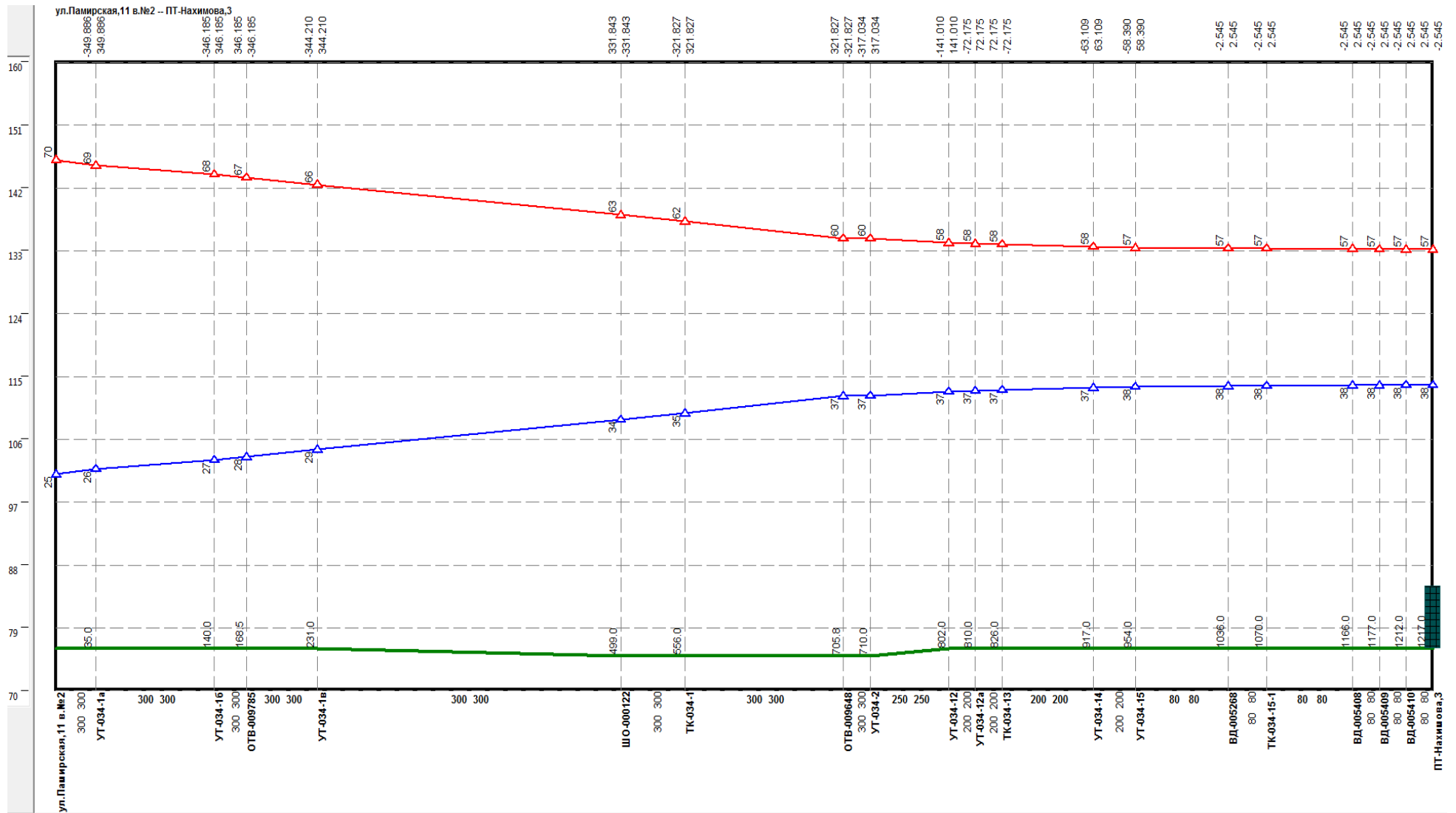
Рисунок 0.16 –Результат гидравлического расчета - график гидравлических режимов по пути теплоносителя от ТЭС-3 до ПТ-Нахимова,3
