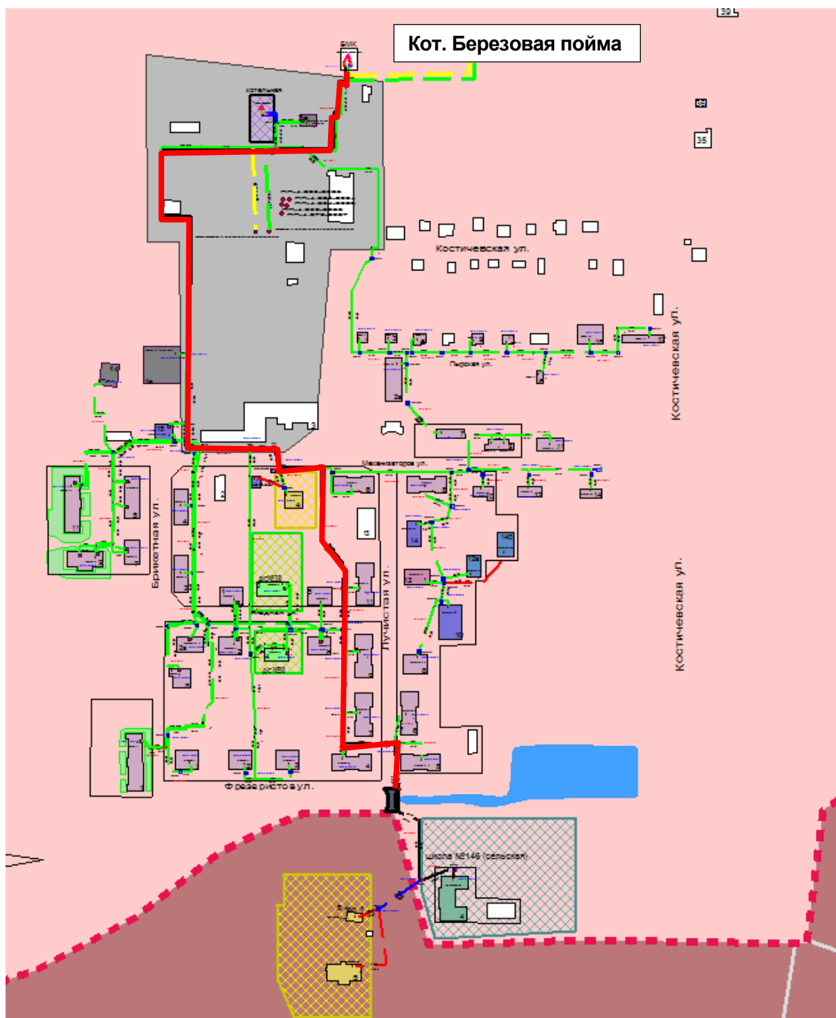
Рисунок 0.97 – Результат гидравлического расчета - расчетный путь теплоносителя от котельной Березовая пойма до ПТ-Лучистая,4
