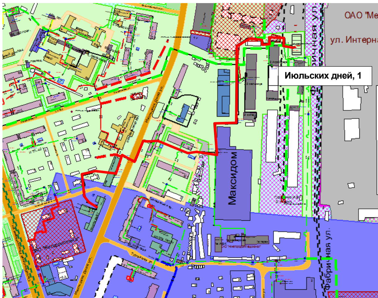
Рисунок 0.103 – Результат гидравлического расчета - расчетный путь теплоносителя от Июльских дней, 1 до ПТ-Июльских дней, 10 школа
