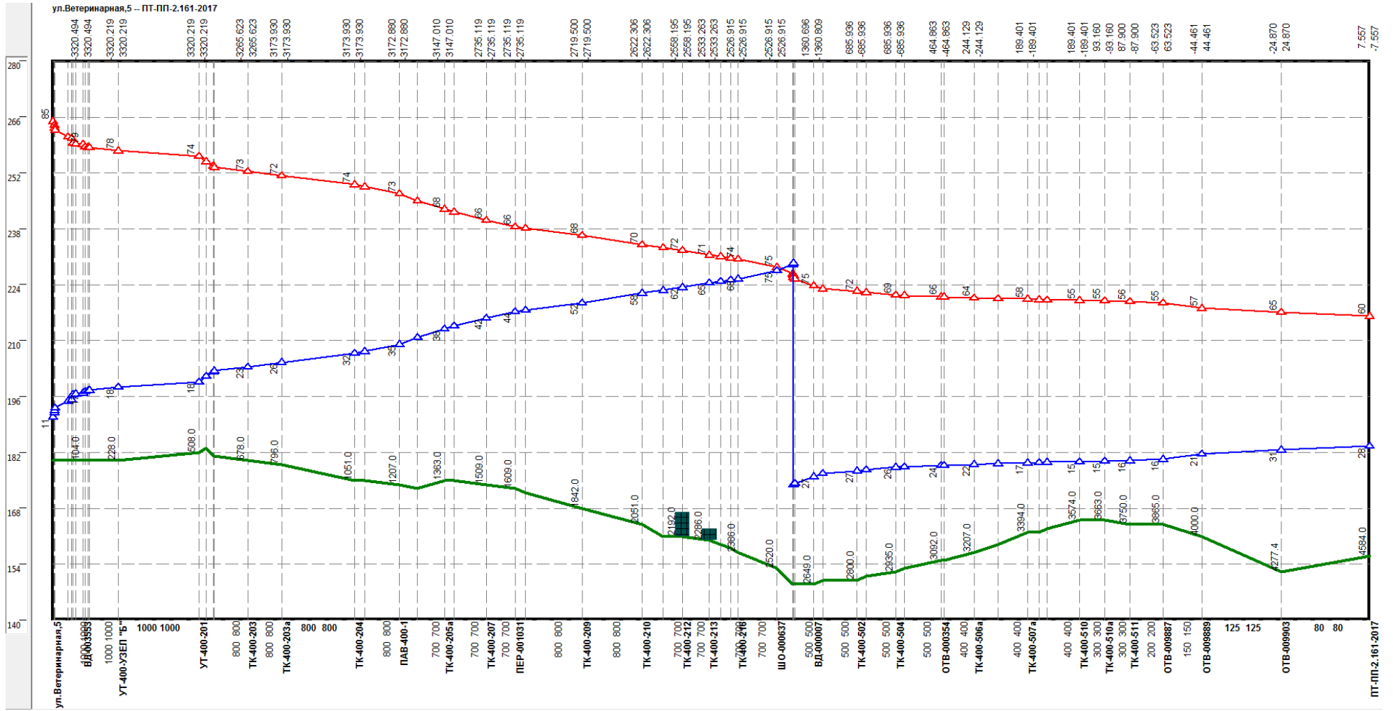
Рисунок 0.120 –Результат гидравлического расчета - график гидравлических режимов по пути теплоносителя от котельной НТЦ до ОТВ-009903
