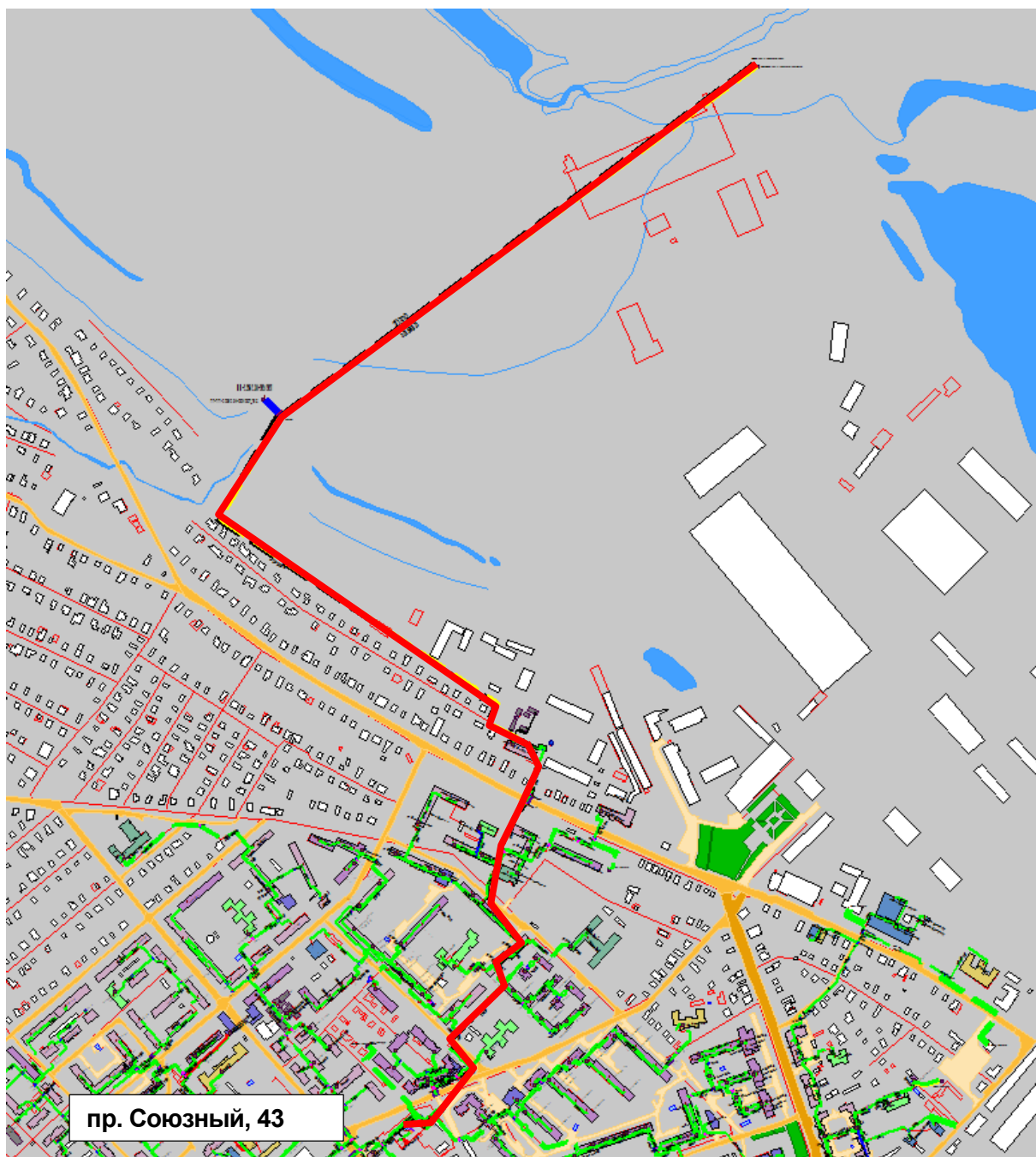
Рисунок 0.73 – Результат гидравлического расчета - расчетный путь теплоносителя от котельной пр. Союзный, 43 до ПТ-ПП-4.101/1.182-2018/2027
