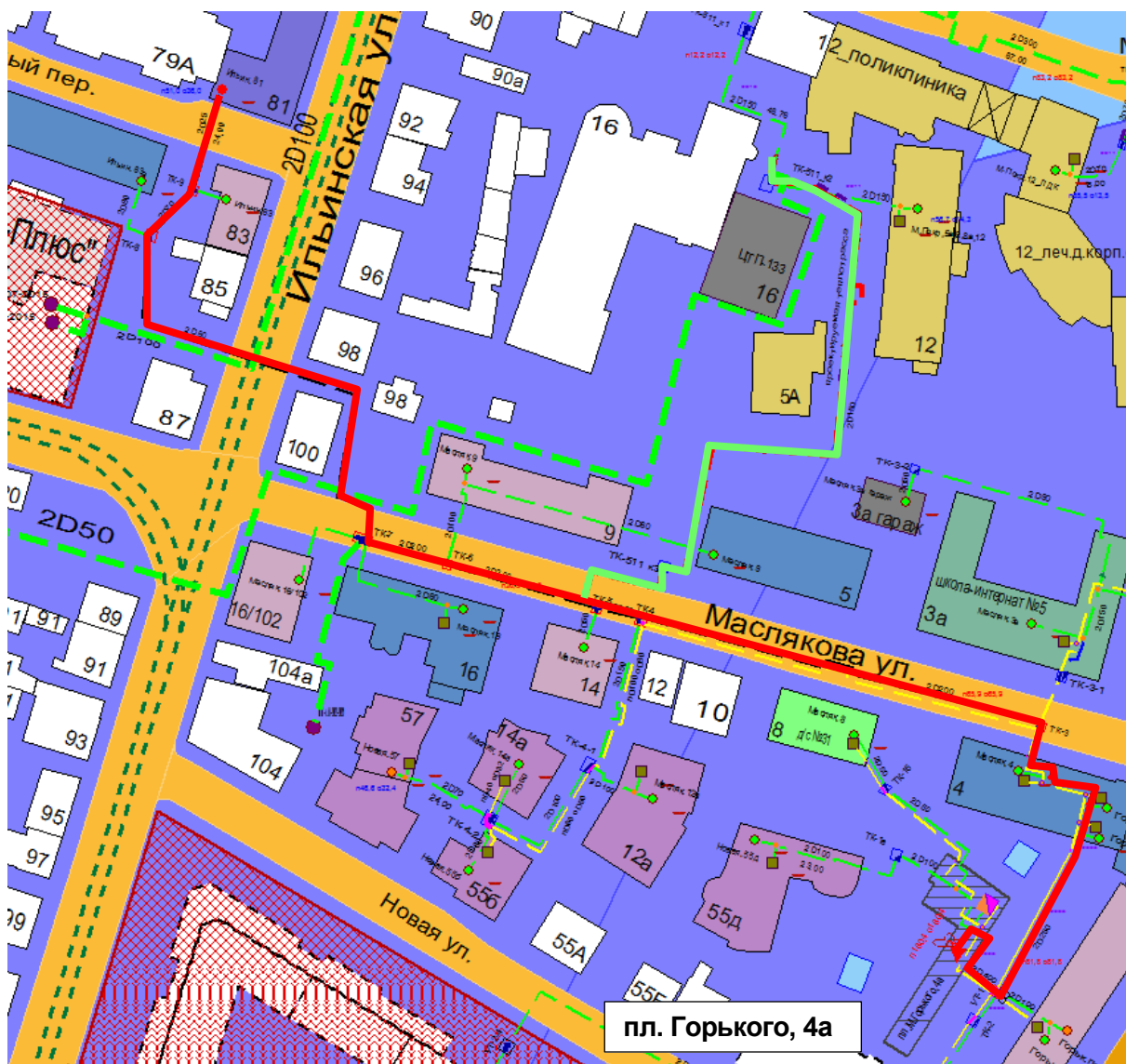
Рисунок 0.71 – Результат гидравлического расчета - расчетный путь теплоносителя от котельной пл. Горького, 4а до ПТ-Ильин,81
