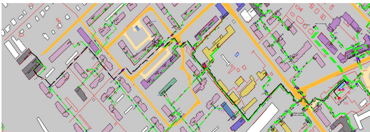
Рисунок 0.131 - Результат гидравлического расчета - расчетный путь теплоносителя от котельной пр. Союзный, 43 до ПТ-Комин,256 э2
