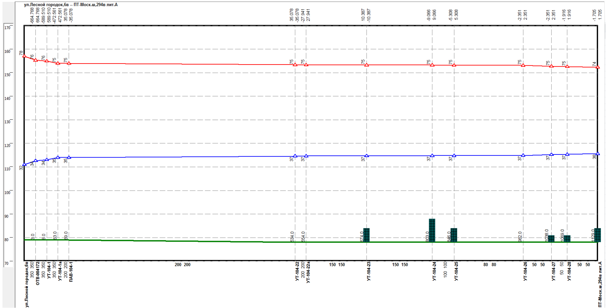
Рисунок 0.20 –Результат гидравлического расчета - график гидравлических режимов по пути теплоносителя от Лесной городок, 6в до ПТ-Моск.ш,294в лит.А
