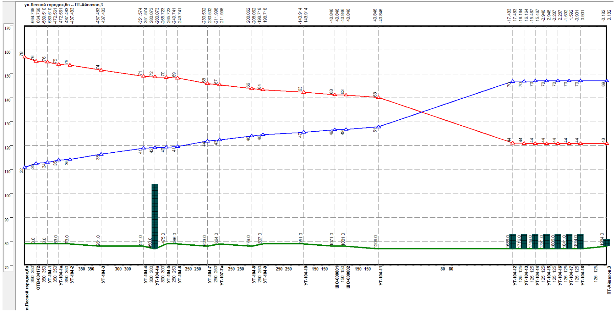
Рисунок 0.18 –Результат гидравлического расчета - график гидравлических режимов по пути теплоносителя от Лесной городок, 6в до ПТ-Айвазов,3
