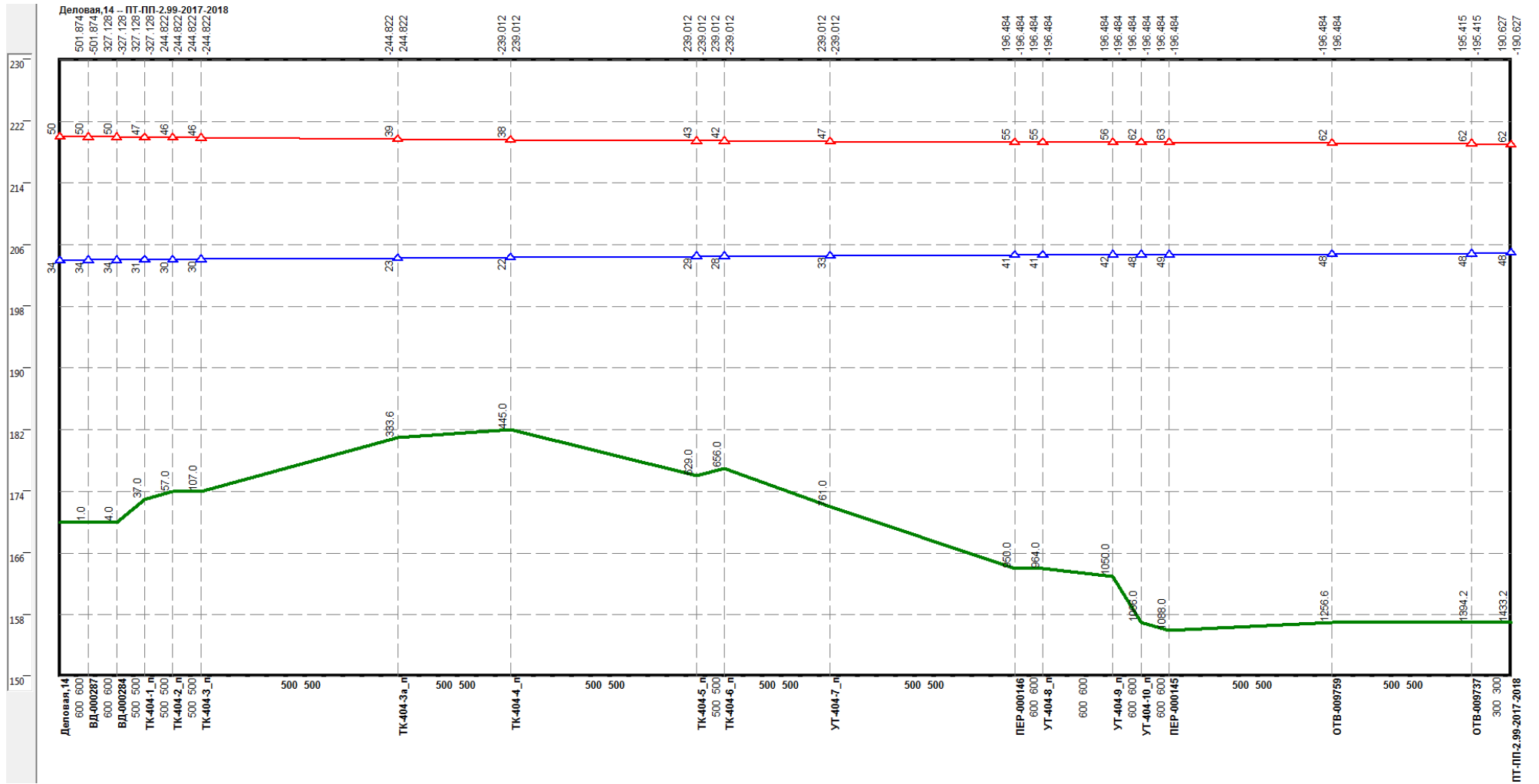
Рисунок 0.102 –Результат гидравлического расчета - график гидравлических режимов по пути теплоносителя от котельной Деловая, 14 до ПТ-ПП-2.99-2017-2018.
