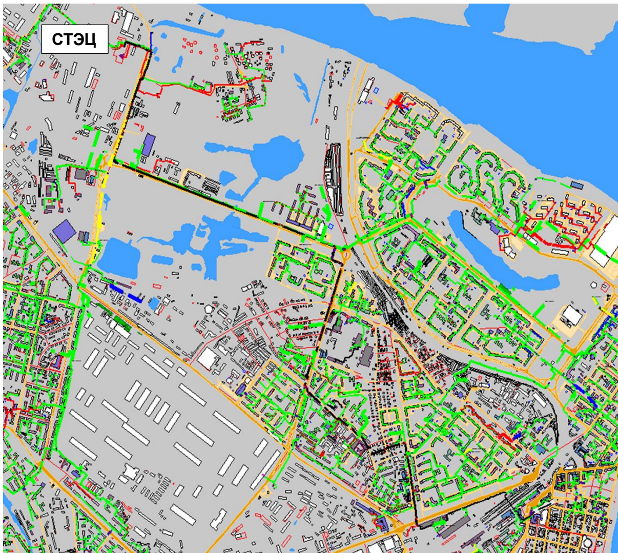
Рисунок 0.87 - Результат гидравлического расчета - расчетный путь теплоносителя от СТЭЦ до ПТ-пл.Револ,7 вест2
