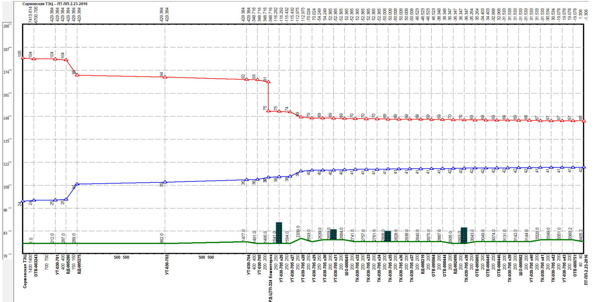
Рисунок 0.90 –Результат гидравлического расчета - график гидравлических режимов по пути теплоносителя от СТЭЦ до ПТ-ПП-2.23-2016
