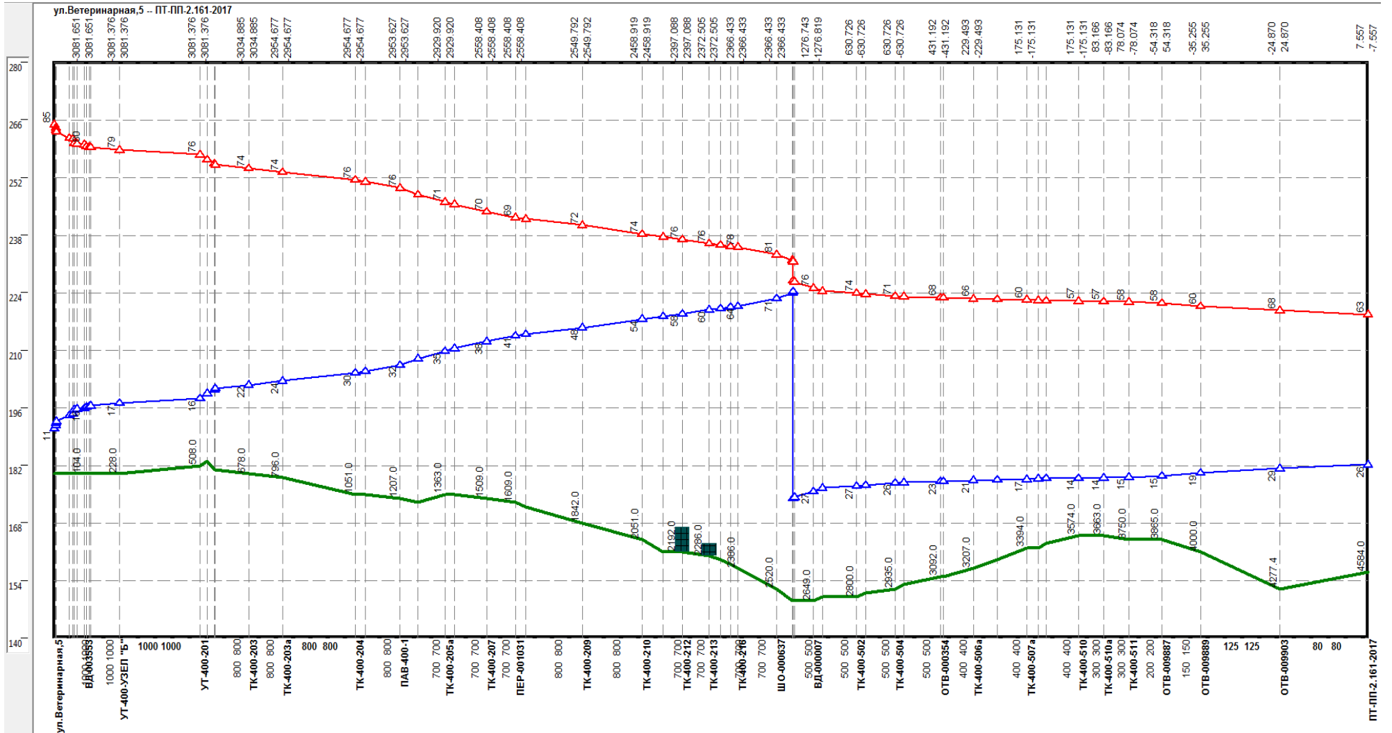
Рисунок 0.64 –Результат гидравлического расчета - график гидравлических режимов по пути теплоносителя от котельной НТЦ до ОТВ-009903
