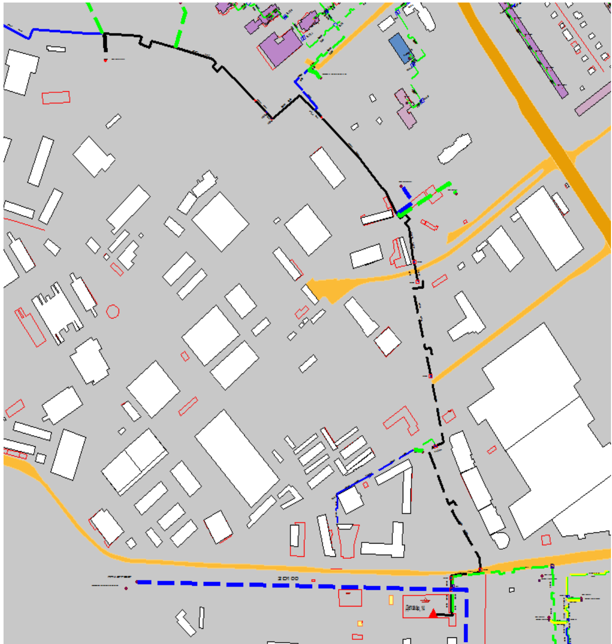
Рисунок 0.101 – Результат гидравлического расчета - расчетный путь теплоносителя от котельной Деловая, 14 до ПТ-ПП-2.99-2017-2018
