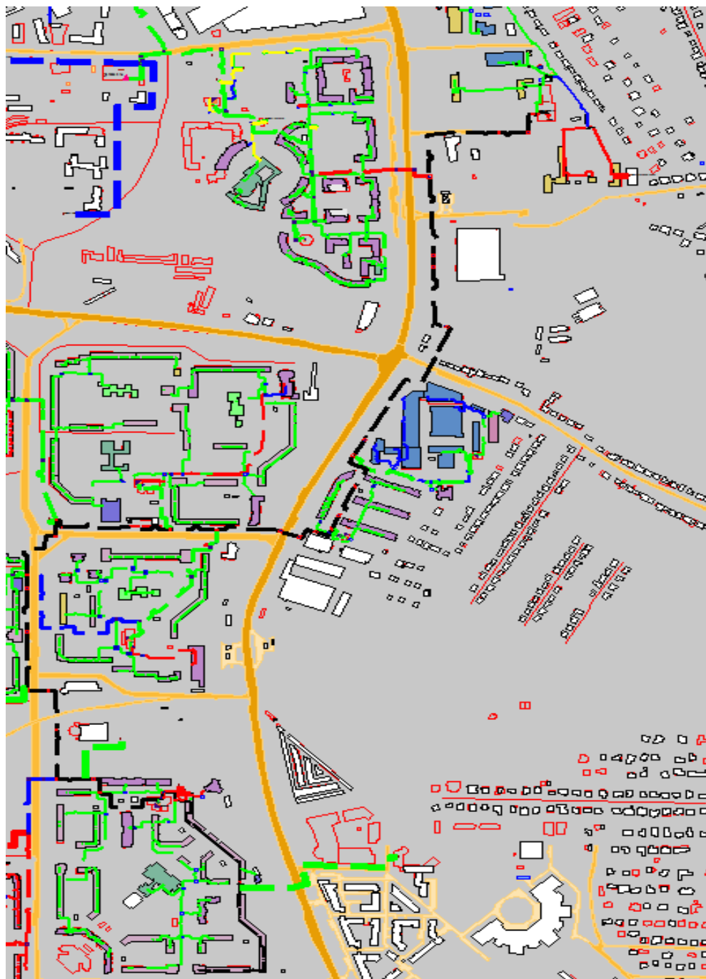
Рисунок 0.79 – Результат гидравлического расчета - расчетный путь теплоносителя от котельной ул. Родионова, 1946 до ПТ-Богдан, 1 пр.
