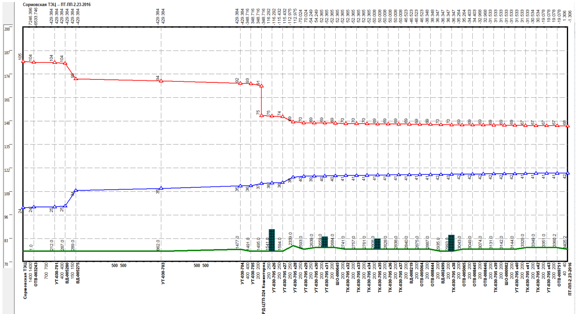
Рисунок 0.8 –Результат гидравлического расчета - график гидравлических режимов по пути теплоносителя от СТЭЦ до ПТ-ПП-2.23-2016
