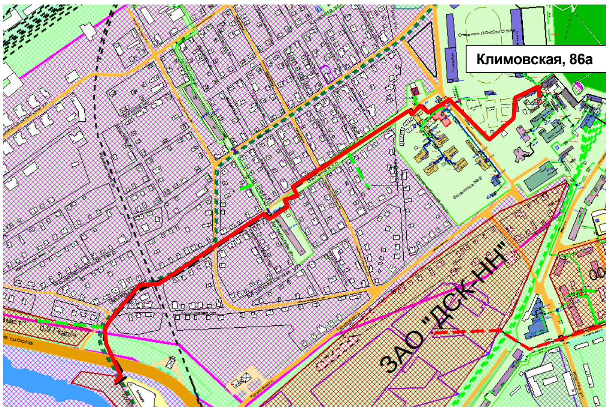
Рисунок 0.113 – Результат гидравлического расчета - расчетный путь теплоносителя от котельной Климовская, 86а до ПТ-ПП-2.227-2016
