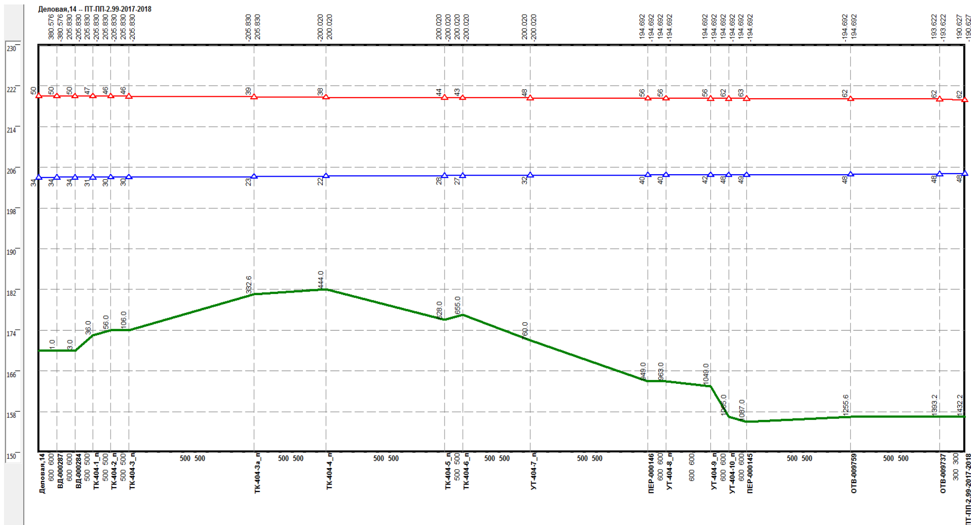
Рисунок 0.30 –Результат гидравлического расчета - график гидравлических режимов по пути теплоносителя от котельной Деловая, 14 до ПТ-ПП-2.99-2017-2018.
