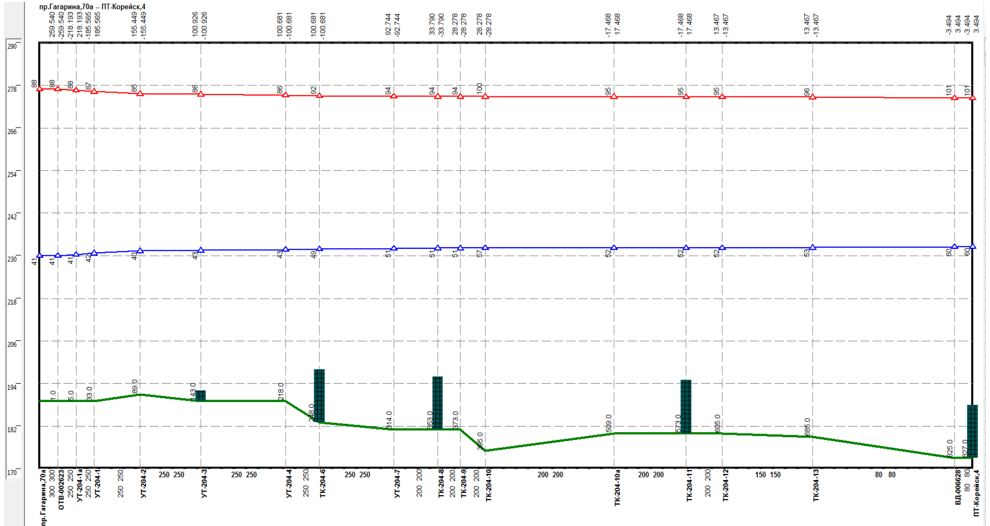
Рисунок 0.56 –Результат гидравлического расчета - график гидравлических режимов по пути теплоносителя от котельной пр. Гагарина, 70а до ПТ-Корейск,4
