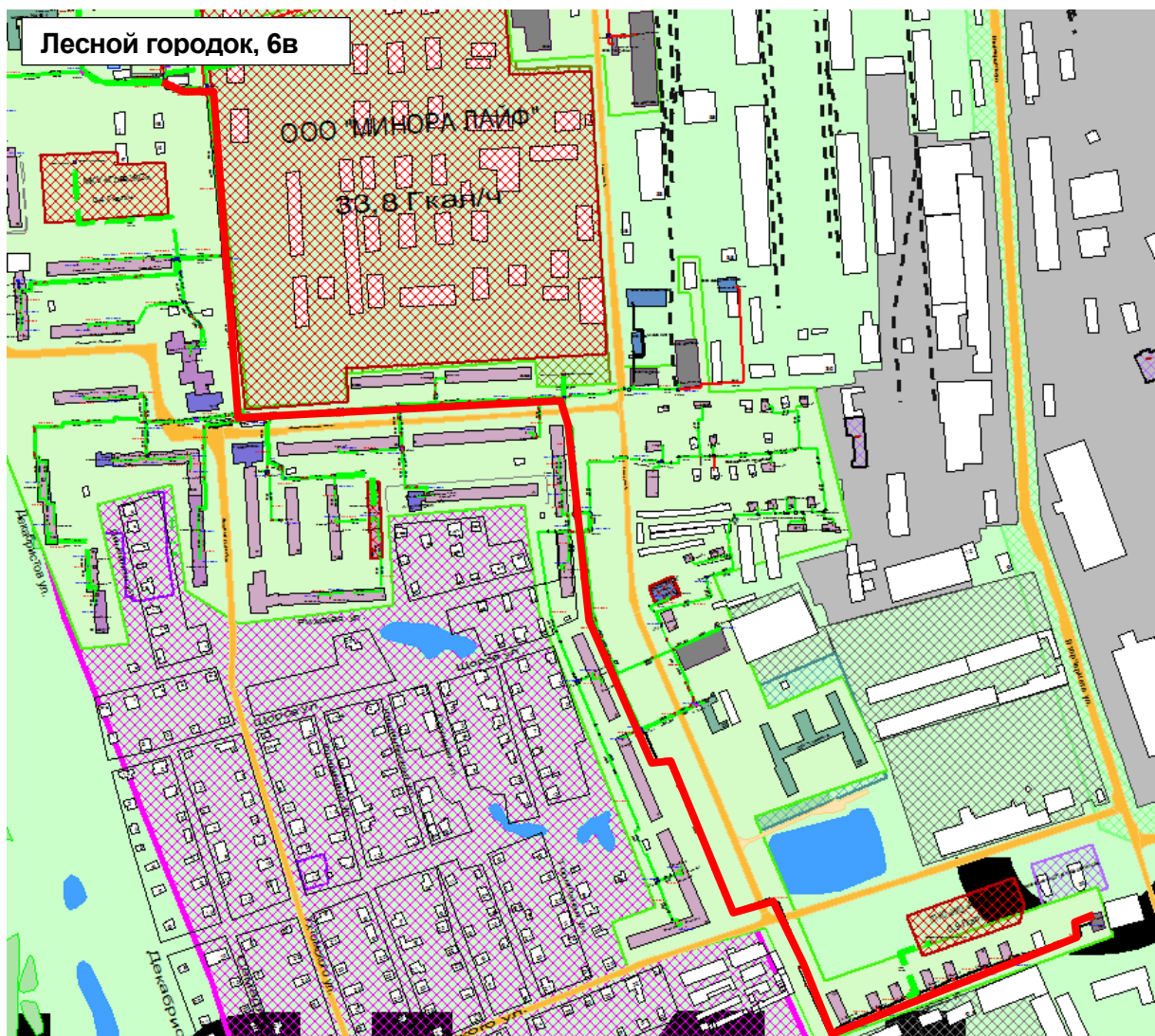
Рисунок 0.17 – Результат гидравлического расчета - расчетный путь теплоносителя от Лесной городок, 6в до ПТ-Айвазов,3
