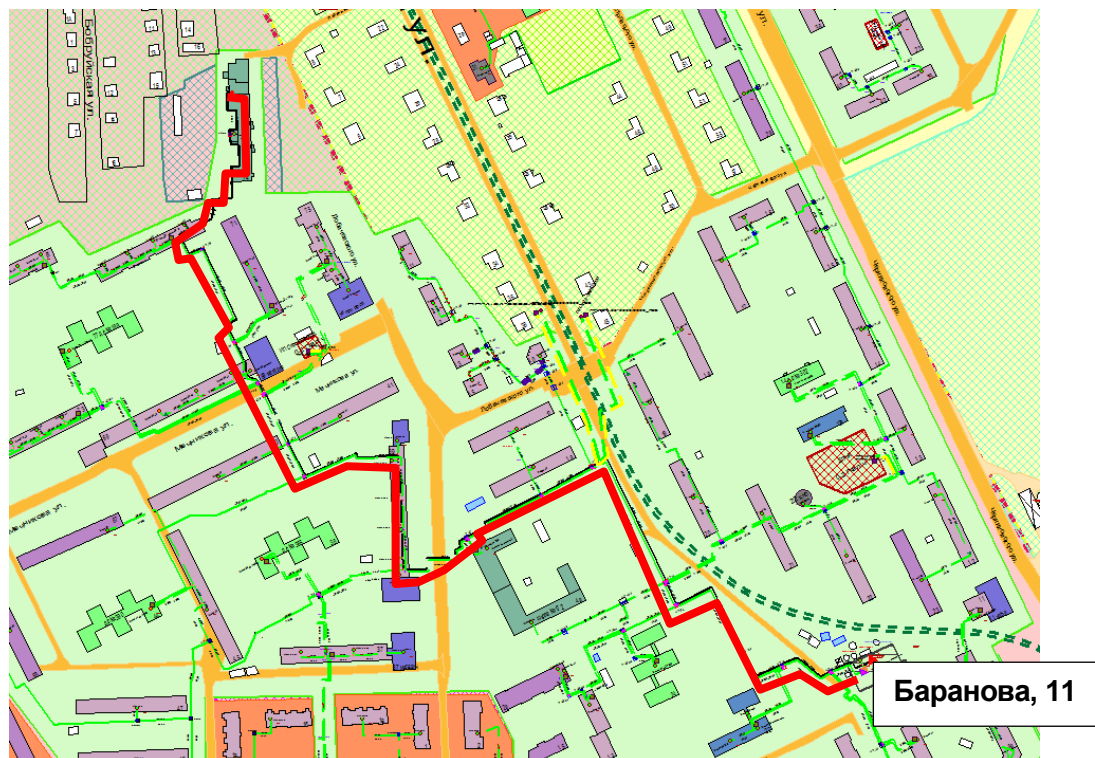
Рисунок 0.107 – Результат гидравлического расчета - расчетный путь теплоносителя от котельной Баранова, 11 до ПТ-Мечн, 74 маст
