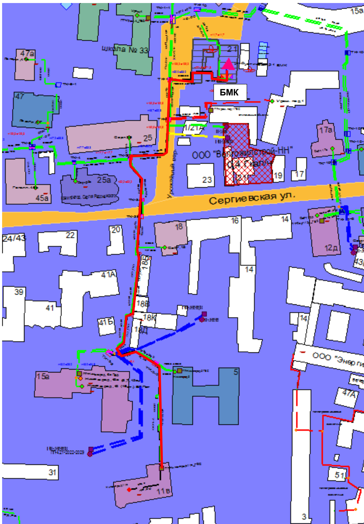
Рисунок 0.9 – Результат гидравлического расчета - расчетный путь теплоносителя от котельной Суетинская, 21 до ПТ-Нтжегород,11в
