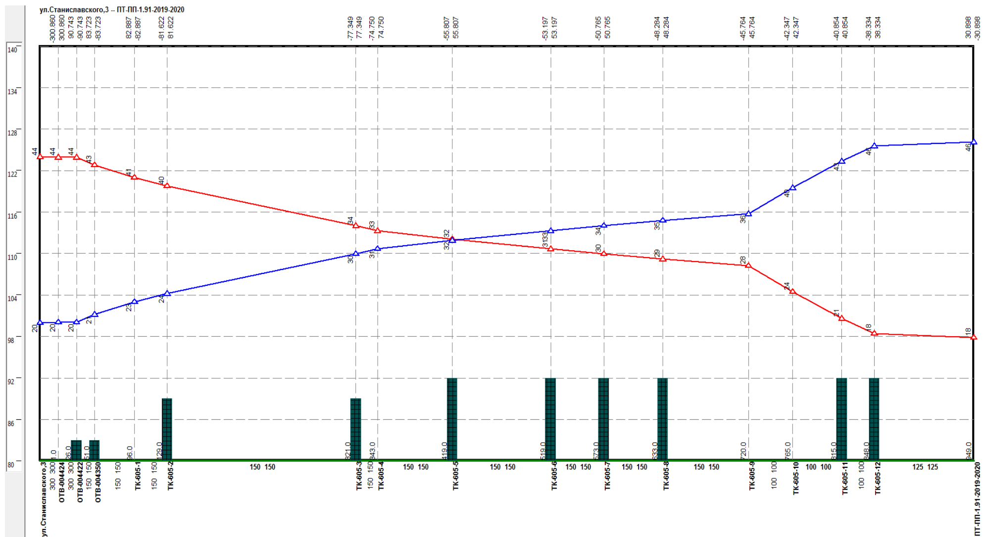
Рисунок 0.48 –Результат гидравлического расчета - график гидравлических режимов по пути теплоносителя от котельной Станиславского, 3 до ПТ- ПП-1,91-2019-2020.
