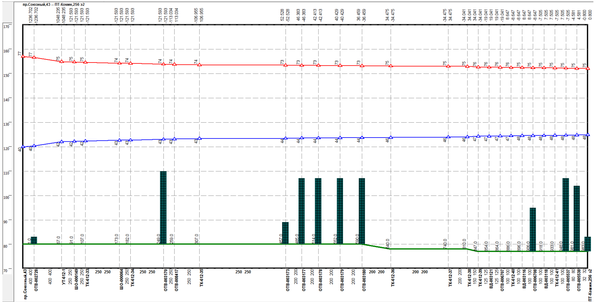
Рисунок 0.132 –Результат гидравлического расчета - график гидравлических режимов по пути теплоносителя от котельной пр. Союзный, 43 до ПТ-Комин,256 э2
