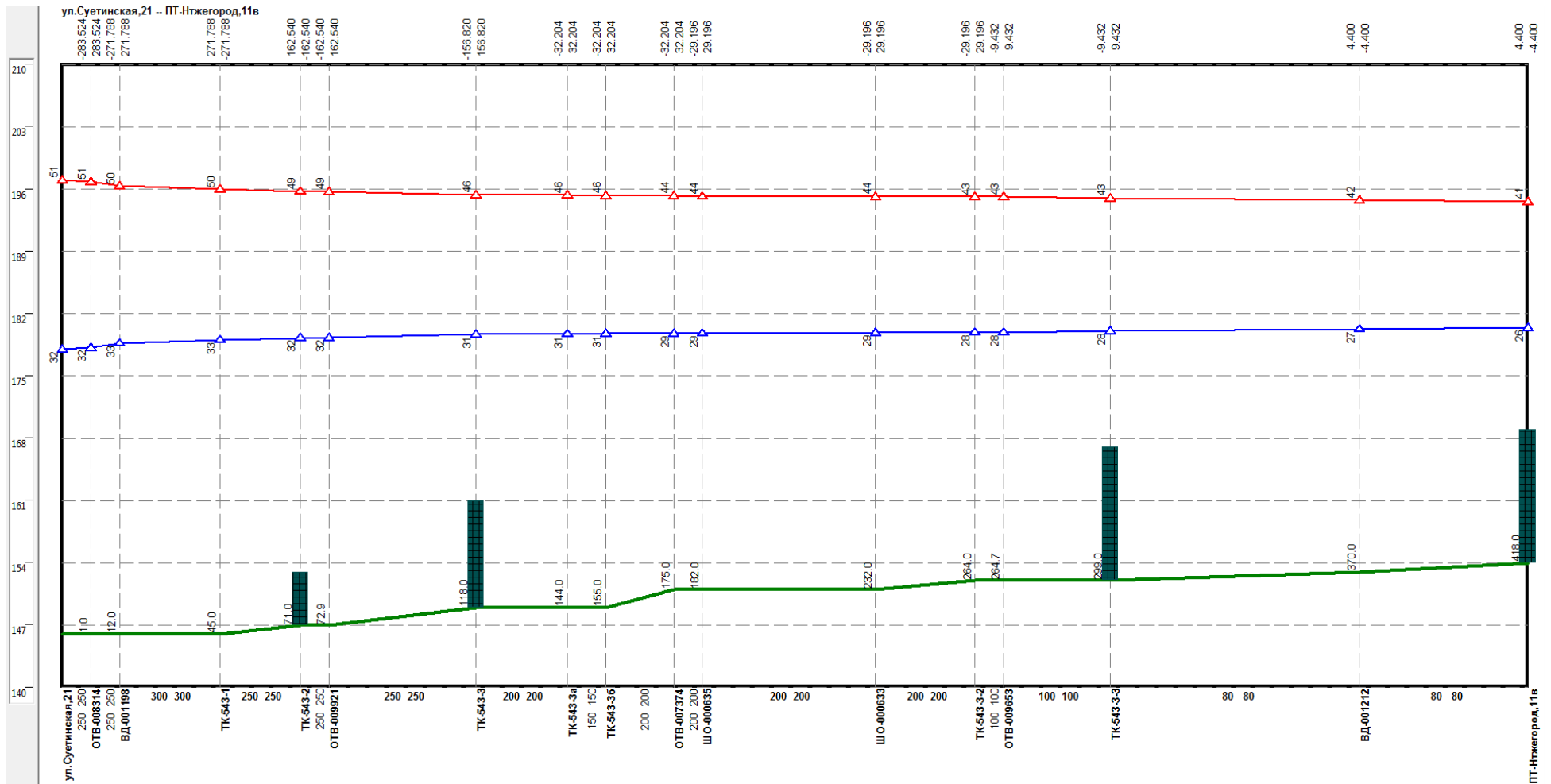
Рисунок 0.10 –Результат гидравлического расчета - график гидравлических режимов по пути теплоносителя от котельной Суетинская, 21 до ПТ-Нтжегород,11в
