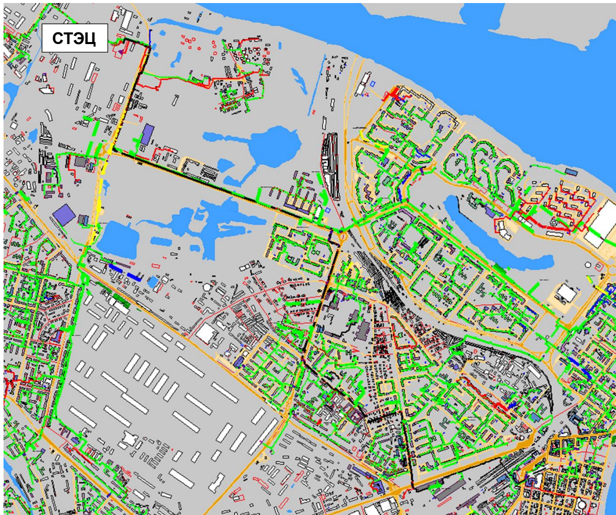
Рисунок 0.5 - Результат гидравлического расчета - расчетный путь теплоносителя от СТЭЦ до ПТ-Сорм.ш,20 э2
