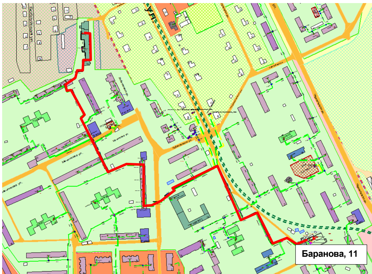
Рисунок 0.39 – Результат гидравлического расчета - расчетный путь теплоносителя от котельной Баранова, 11 до ПТ-Мечн,74 маст
