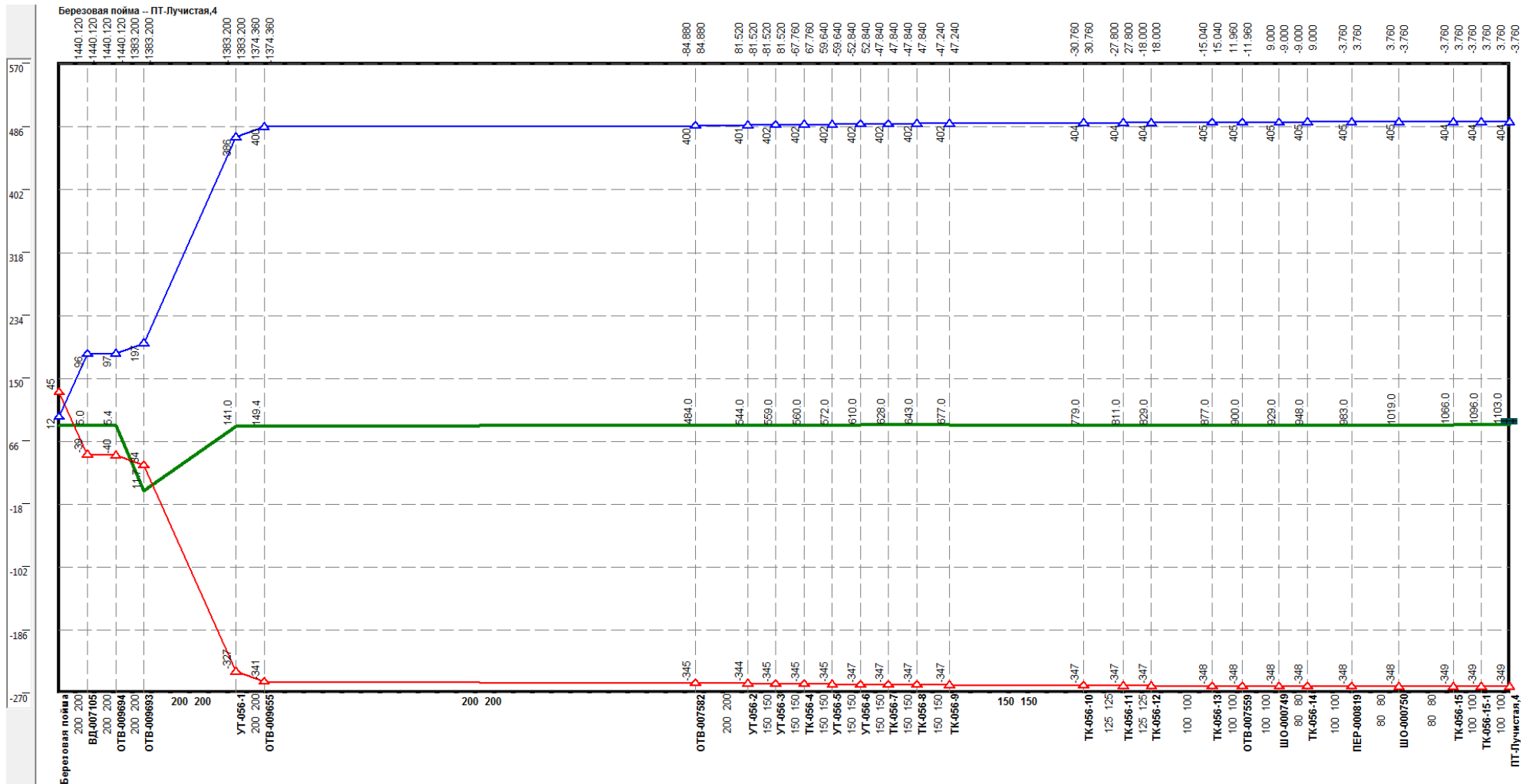
Рисунок 0.98 –Результат гидравлического расчета - график гидравлических режимов по пути теплоносителя от котельной Березовая пойма до ПТ-Лучистая, 4
