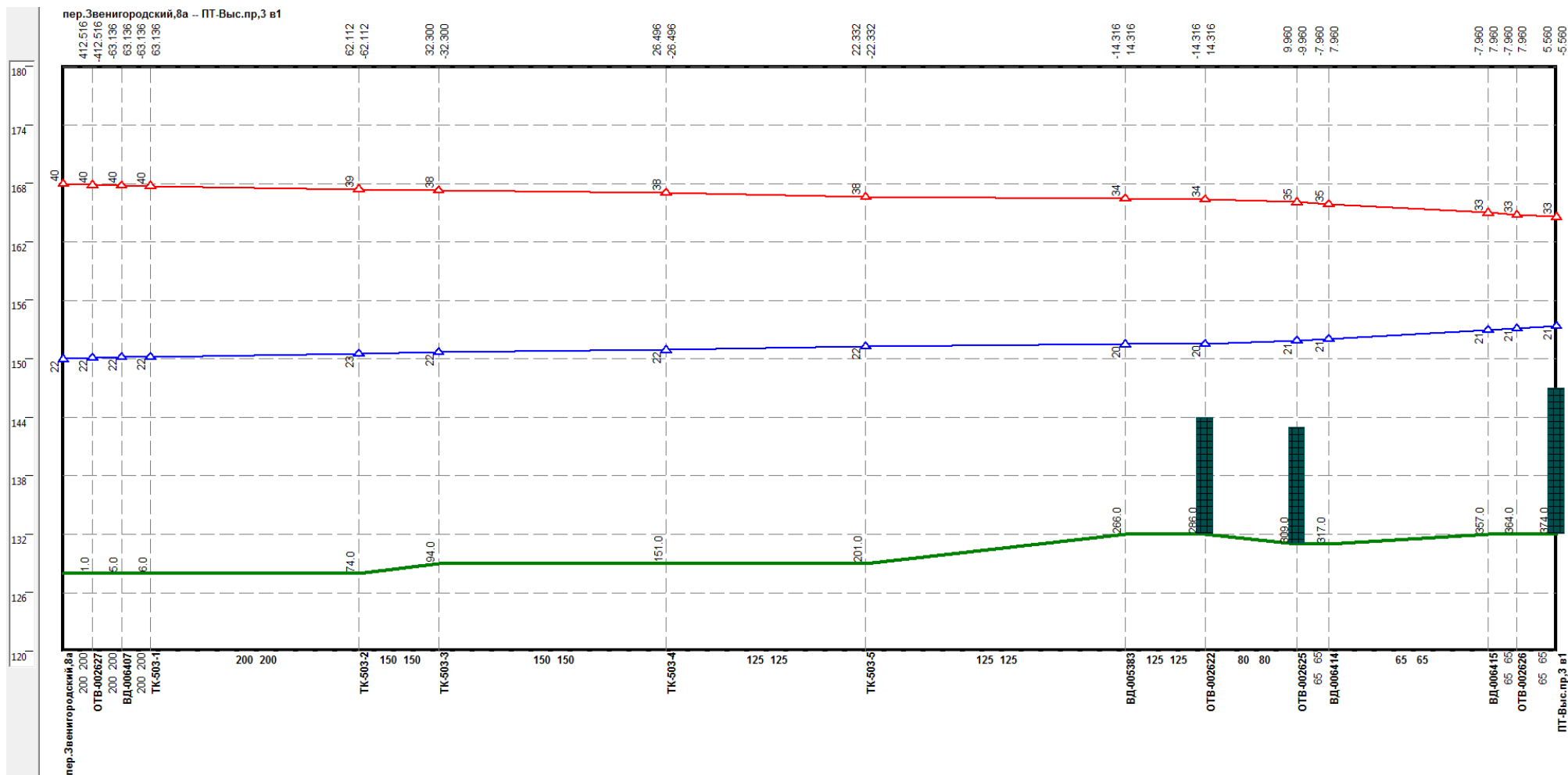
Рисунок 0.52 –Результат гидравлического расчета - график гидравлических режимов по пути теплоносителя от котельной пер. Звенигородский, 8а до ПТ-Выс.пр,3 в1
