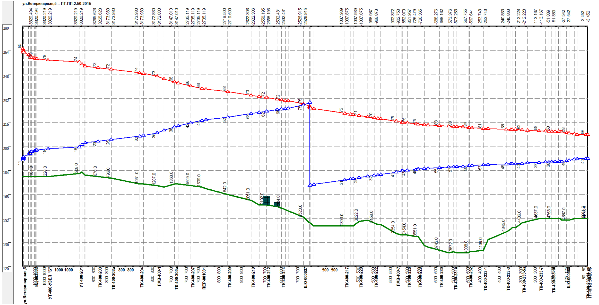
Рисунок 0.118 – Результат гидравлического расчета - график гидравлических режимов по пути теплоносителя от котельной НТЦ до ПТ-В. Волж. наб, проект
