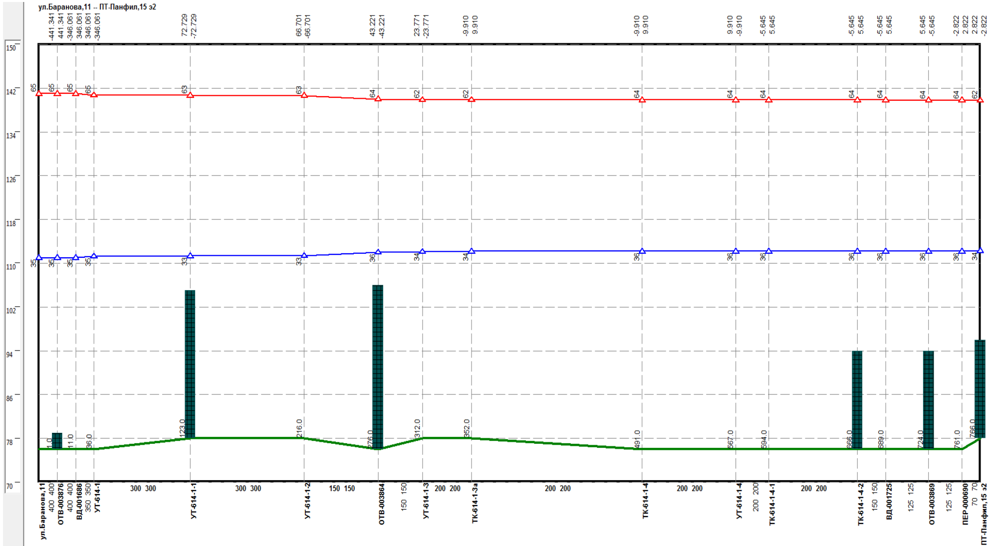
Рисунок 0.42 –Результат гидравлического расчета - график гидравлических режимов по пути теплоносителя от Бойновский, 9д до ПТ-Б.Печер, 93 МВД
