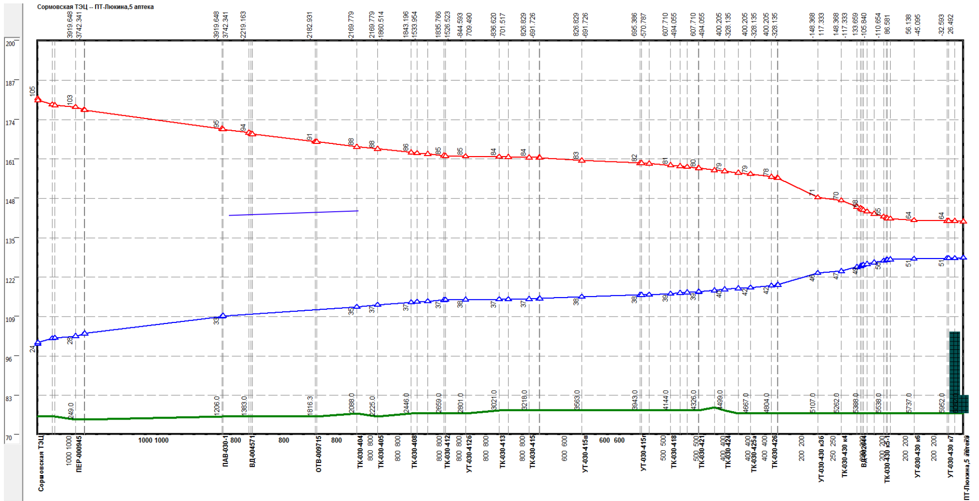
Рисунок 0.84 –Результат гидравлического расчета - график гидравлических режимов по пути теплоносителя от СТЭЦ до ПТ-Люкина,5 аптека
