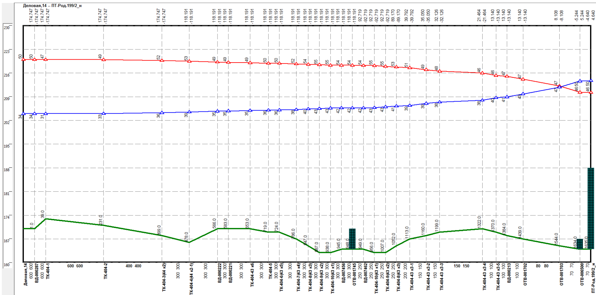
Рисунок 0.100 –Результат гидравлического расчета - график гидравлических режимов по пути теплоносителя от котельной Деловая, 14 до ПТ-Род.199/2_н
