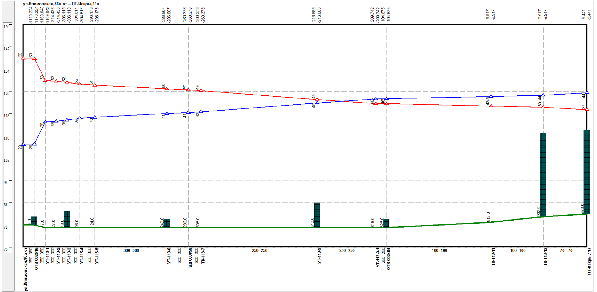
Рисунок 0.44 –Результат гидравлического расчета - график гидравлических режимов по пути теплоносителя от котельной Климовская, 86а до ПТ-Искры,11а
