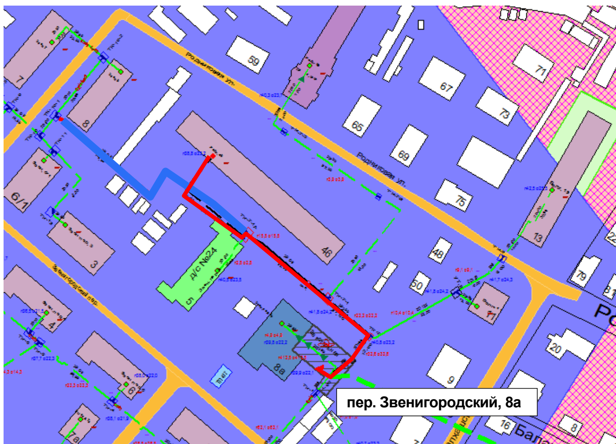
Рисунок 0.53 – Результат гидравлического расчета - расчетный путь теплоносителя от котельной пер. Звенигородский до ПТ-Родн,46
