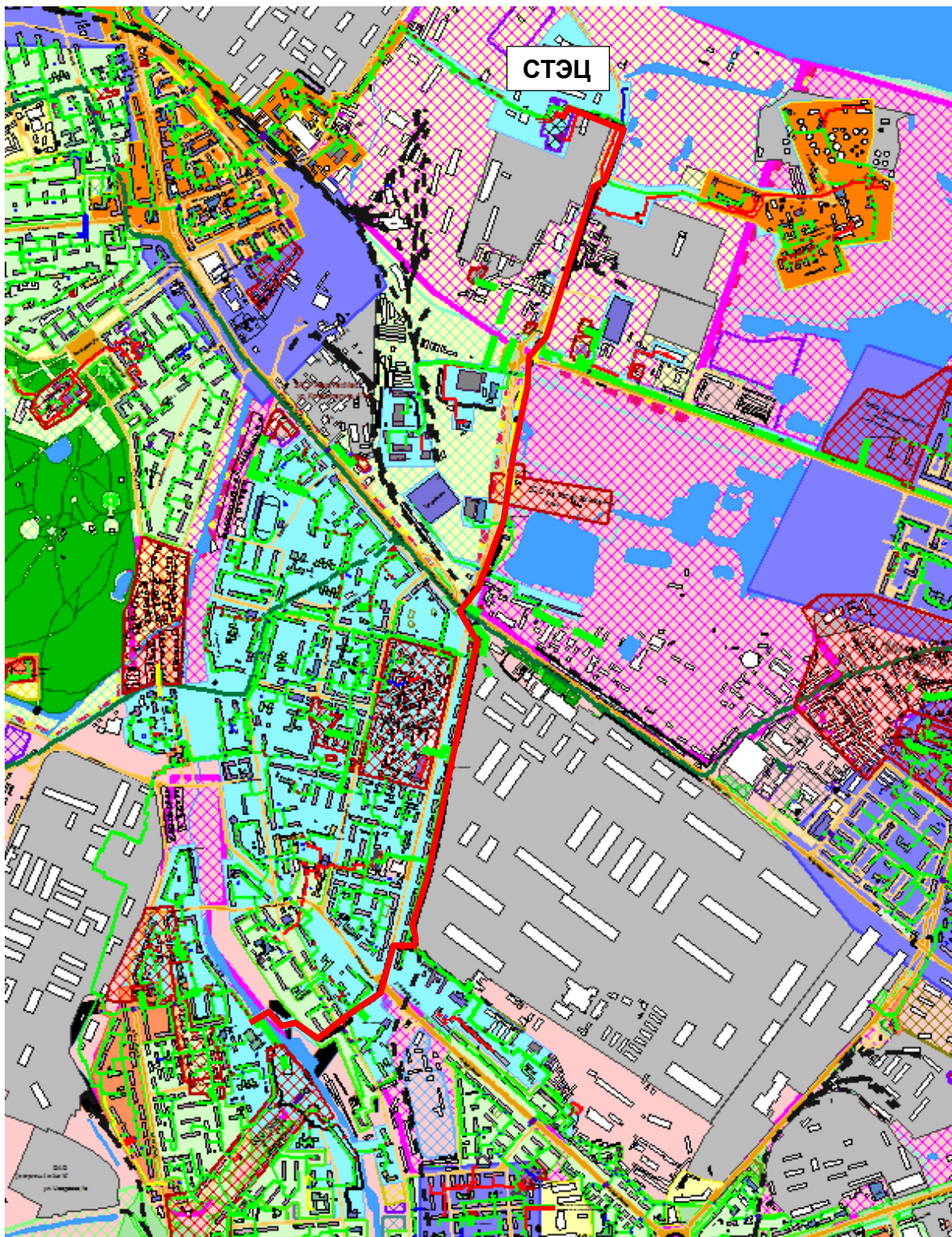
Рисунок 0.83 - Результат гидравлического расчета - расчетный путь теплоносителя от СТЭЦ до ПТ-Люкина,5 аптека
