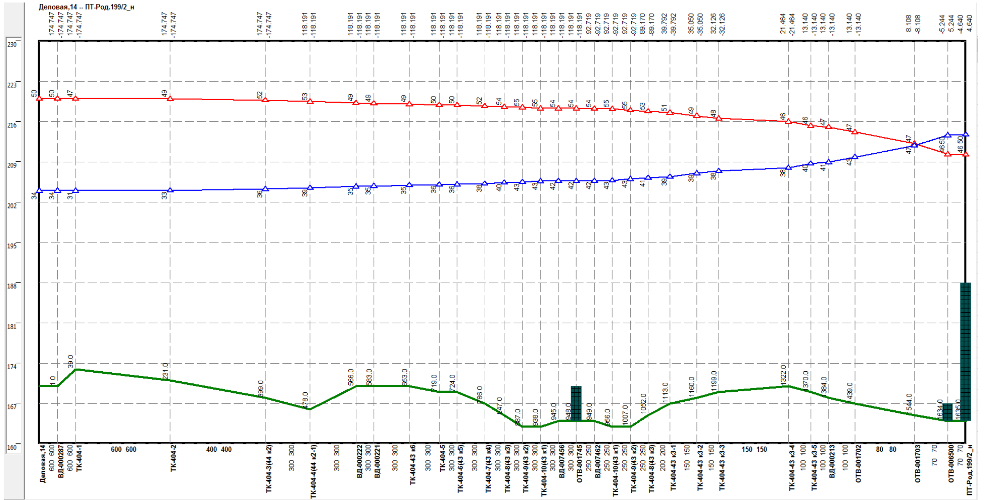
Рисунок 0.28 –Результат гидравлического расчета - график гидравлических режимов по пути теплоносителя от котельной Деловая, 14 до ПТ-Род.199/2_н
