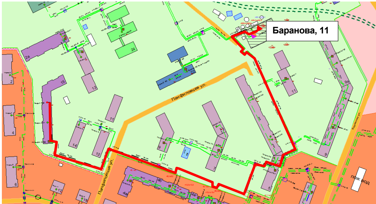
Рисунок 0.109 – Результат гидравлического расчета - расчетный путь теплоносителя от котельной Баранова, 11 до ПТ-Панфил,15 э2
