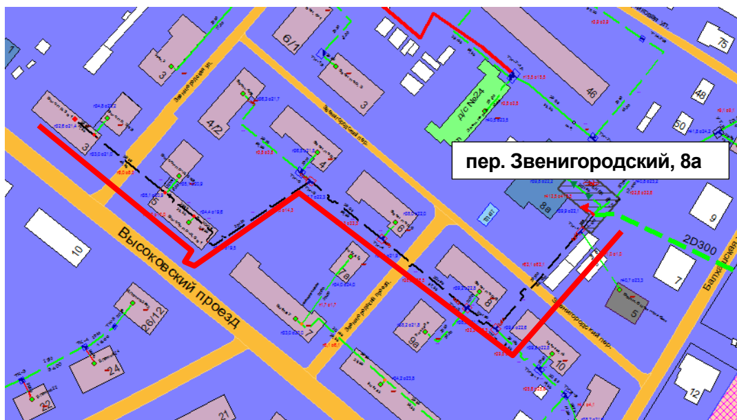
Рисунок 0.51 – Результат гидравлического расчета - расчетный путь теплоносителя от котельной пер. Звенигородский, 8а до ПТ-Выс.пр,3 в1
