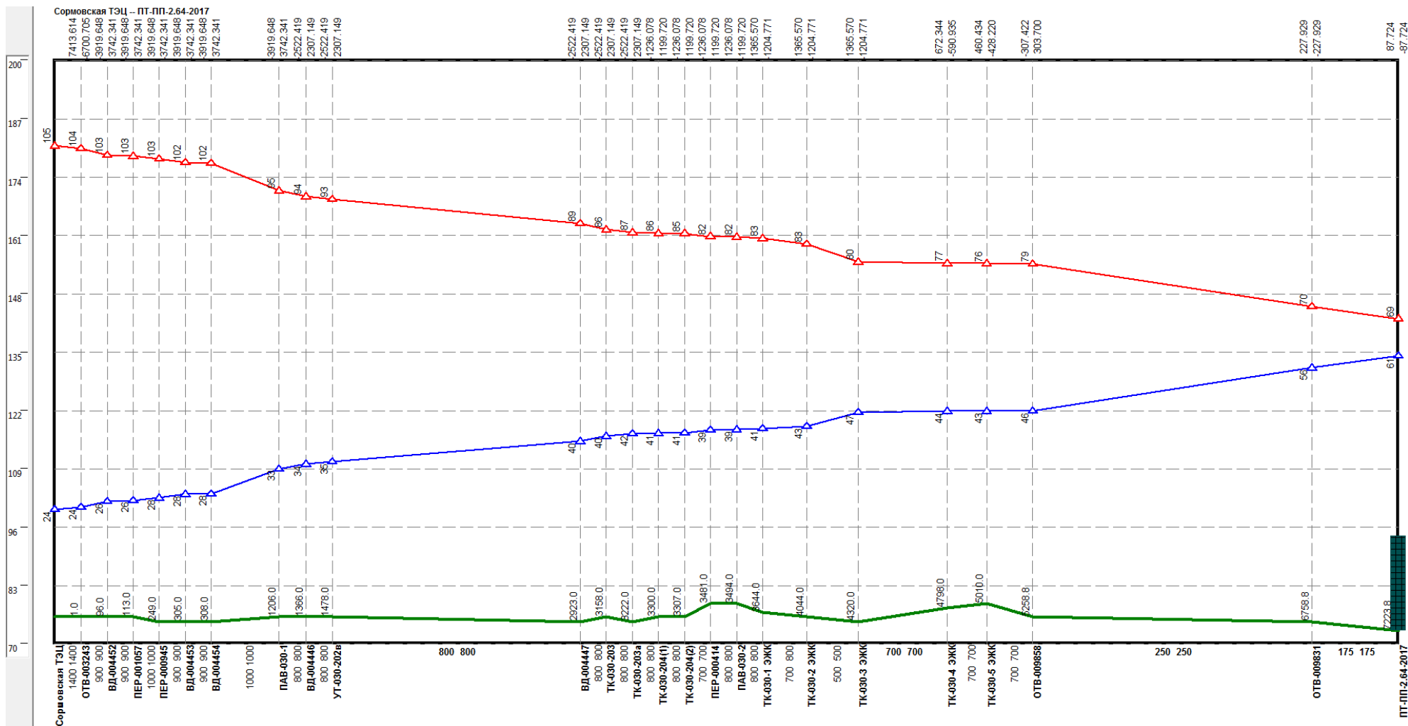
Рисунок 0.86 –Результат гидравлического расчета - график гидравлических режимов по пути теплоносителя от СТЭЦ до ПТ-ПП-2.64-2017
