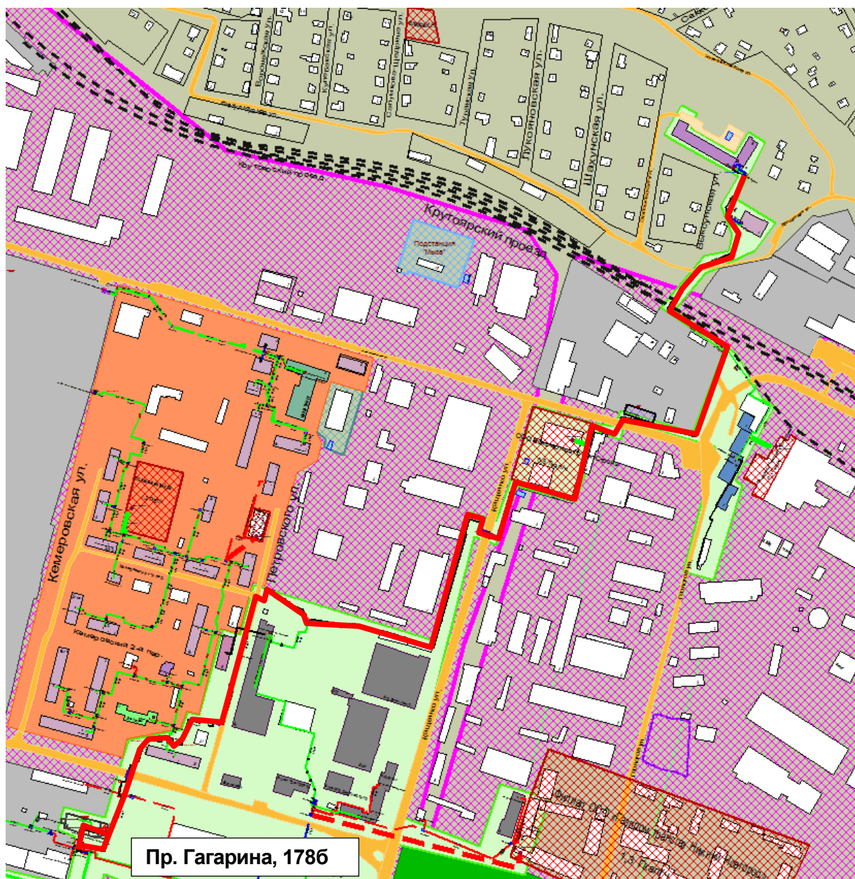
Рисунок 0.67 – Результат гидравлического расчета - расчетный путь теплоносителя от котельной пр. Гагарина, 1786 до ЦТП-706
