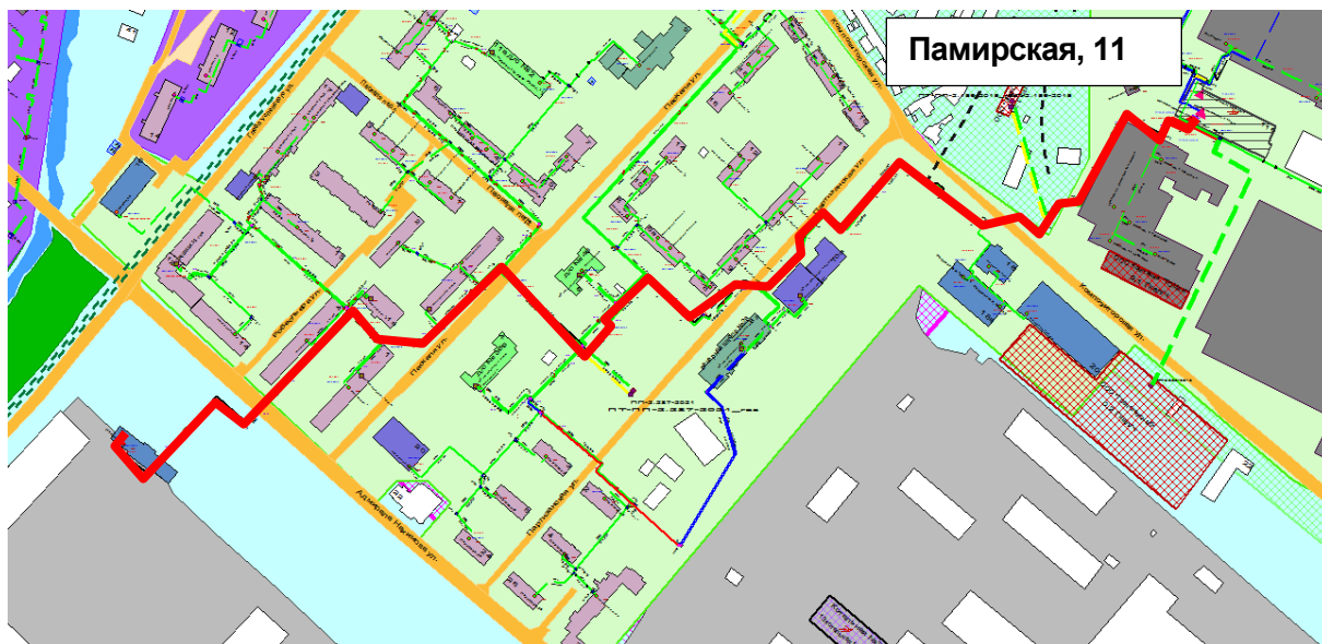
Рисунок 0.15 – Результат гидравлического расчета - расчетный путь теплоносителя от котельной Памирская, 11 до ПТ-Нахимова,3
