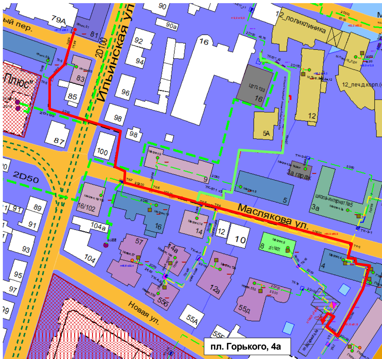
Рисунок 0.127 – Результат гидравлического расчета - расчетный путь теплоносителя от котельной пл. Горького, 4а до ПТ-Ильин,81
