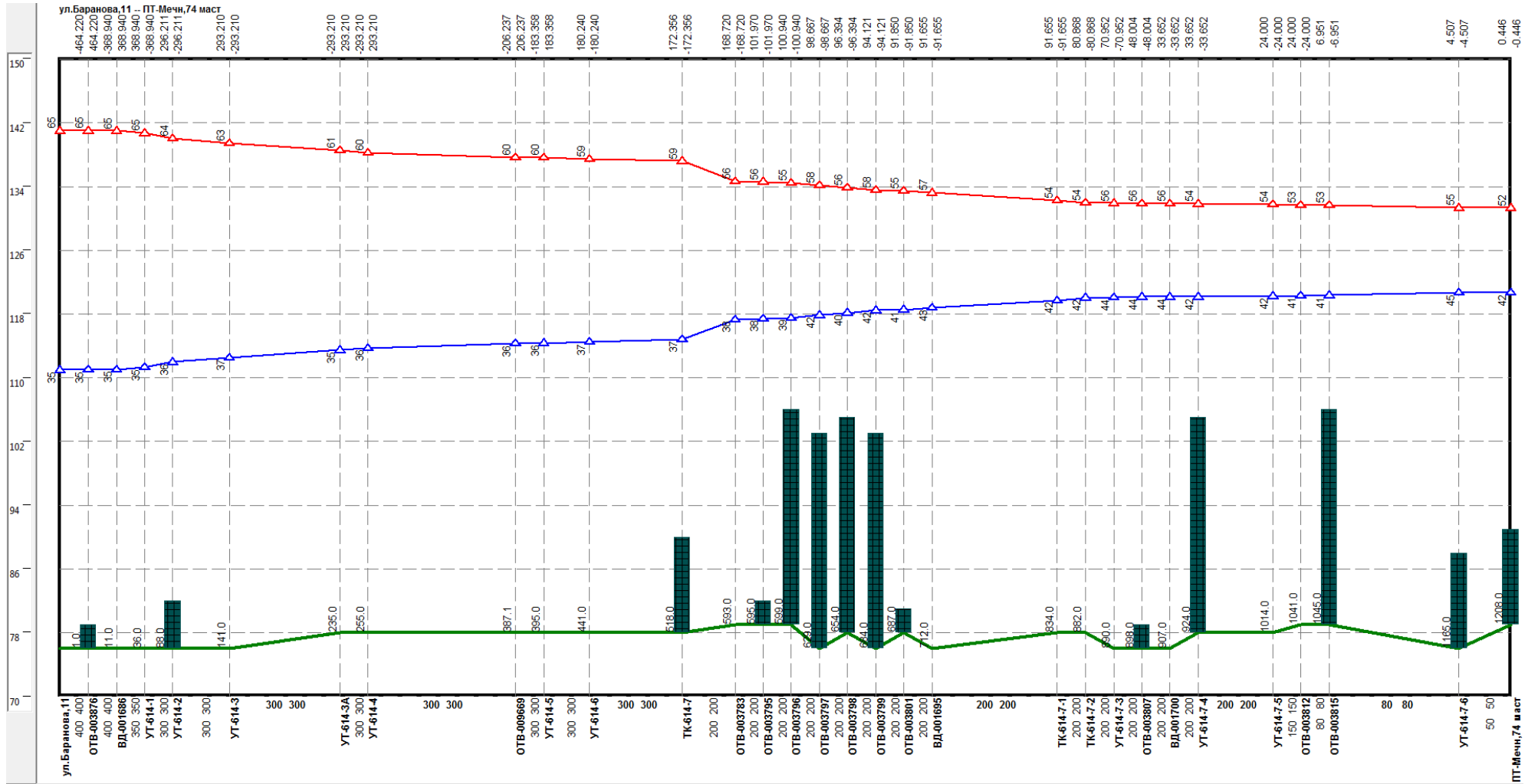
Рисунок 0.108 –Результат гидравлического расчета - график гидравлических режимов по пути теплоносителя от котельной Баранова, 11 до ПТ-Мечн,74 маст
