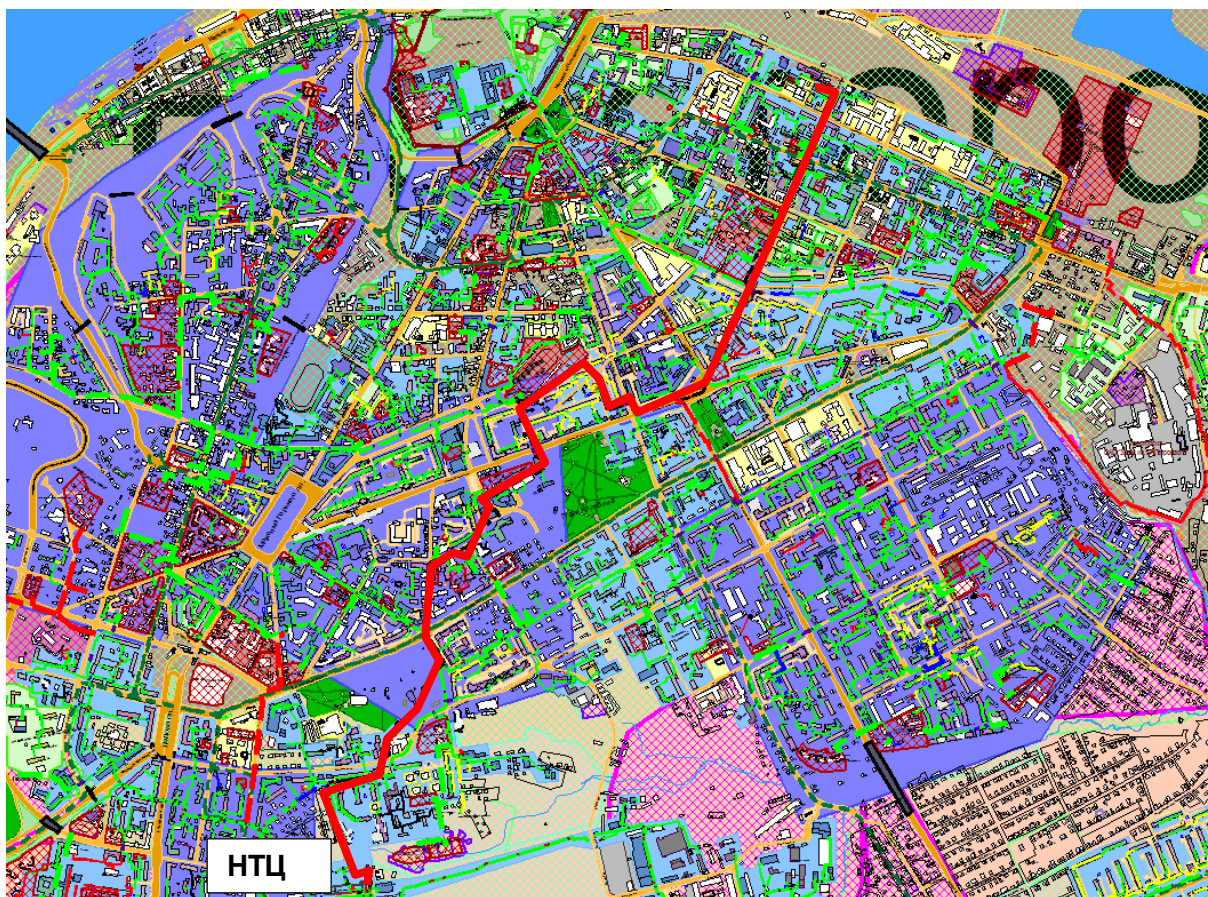
Рисунок 0.117– Результат гидравлического расчета - расчетный путь теплоносителя от котельной НТЦ до ПТ-В.Волж.наб, проект
