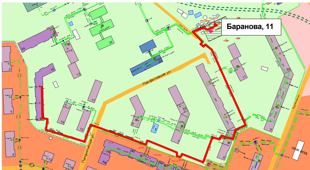
Рисунок 0.41 – Результат гидравлического расчета - расчетный путь теплоносителя от котельной Баранова, 11 до ПТ-Панфил,15 э2
