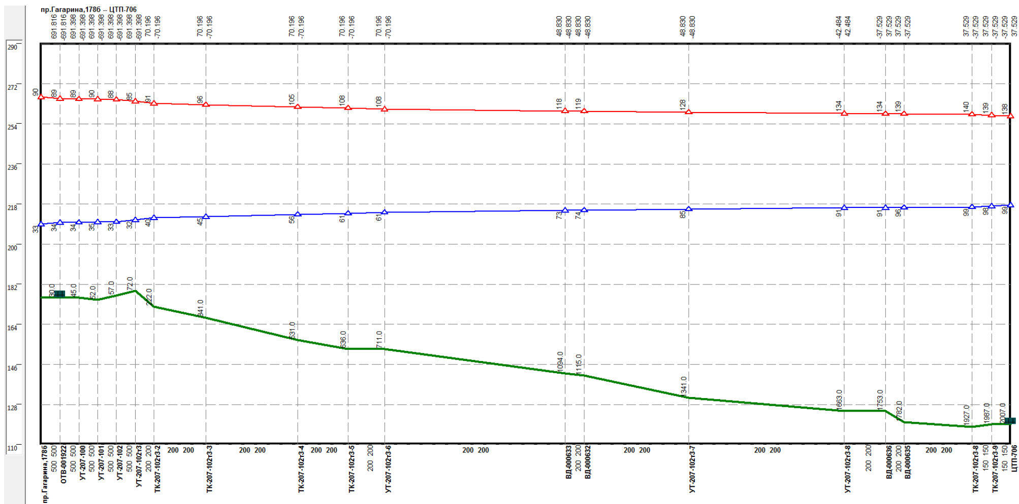
Рисунок 0.68 –Результат гидравлического расчета - график гидравлических режимов по пути теплоносителя от котельной пр. Гагарина, 1786 до ЦТП-706
