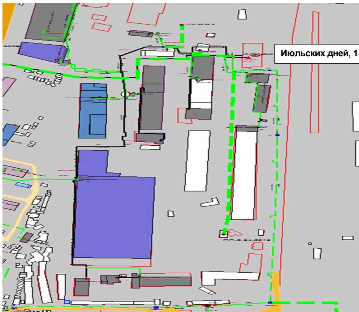
Рисунок 0.105 – Результат гидравлического расчета - расчетный путь теплоносителя от котельной Июльских дней, 1 до ПТ-Деревооб,1а АБК
