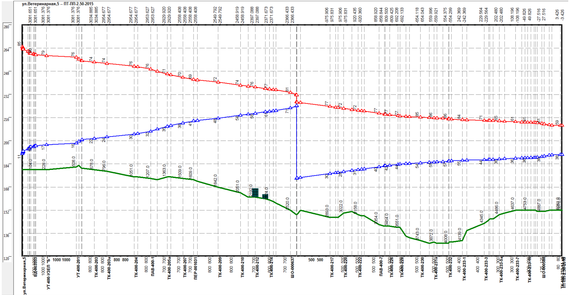
Рисунок 0.62 –Результат гидравлического расчета - график гидравлических режимов по пути теплоносителя от котельной НТЦ до ПТ- ПП-2-50-2015.
