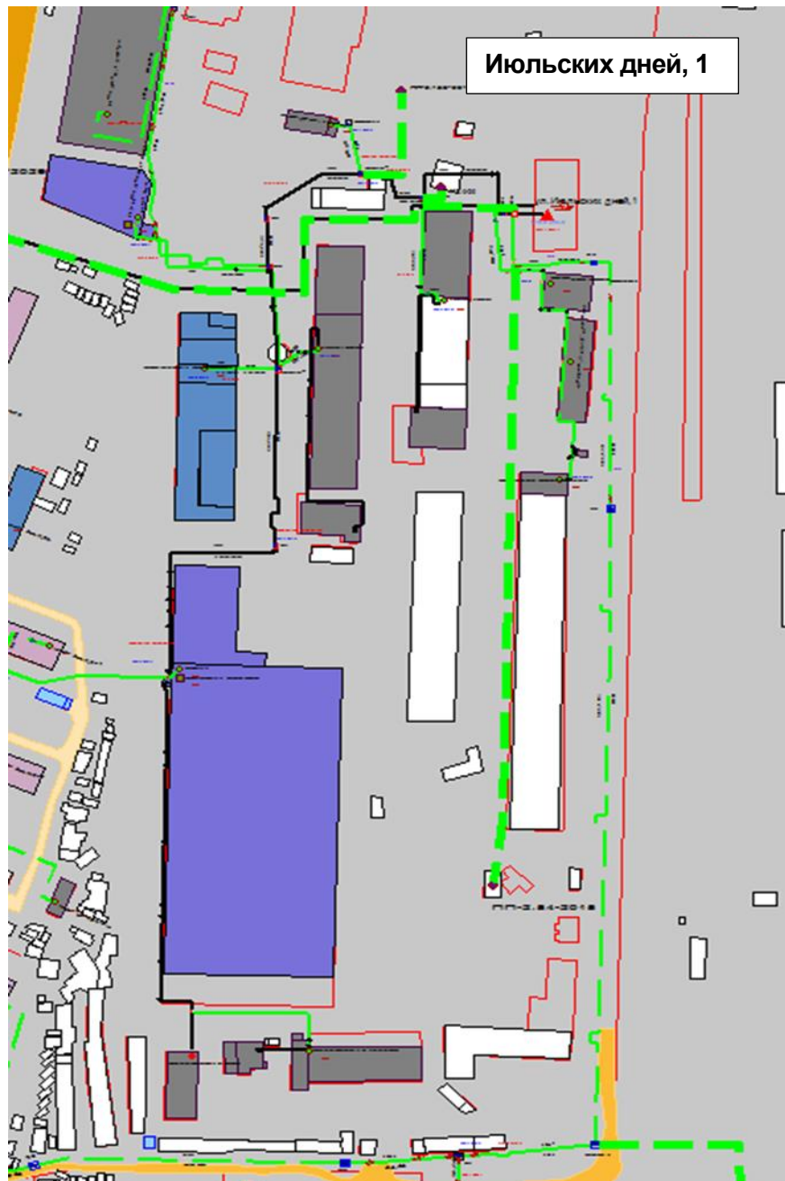
Рисунок 0.33 – Результат гидравлического расчета - расчетный путь теплоносителя от Июльских дней, 1 до ПТ-Деревооб, 1а АБК
