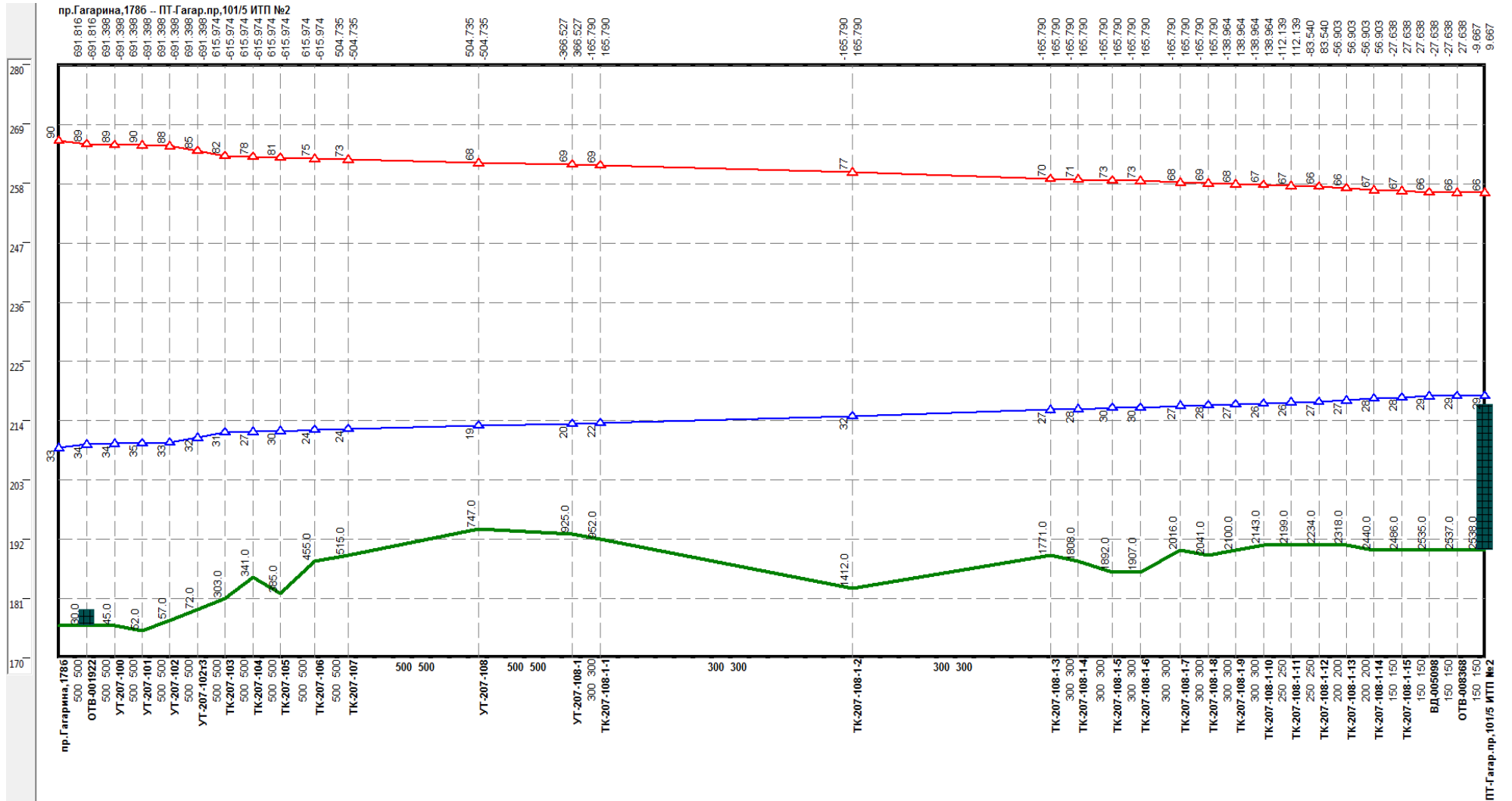
Рисунок 0.70 –Результат гидравлического расчета - график гидравлических режимов по пути теплоносителя от котельной пр. Гагарина, 1786 до ПТ-Гагар.пр.101/5 ИТП №2.
