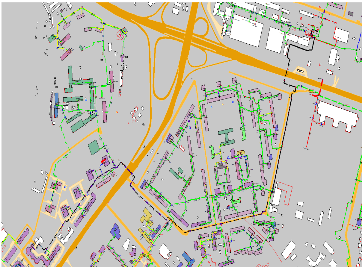
Рисунок 0.125 - Результат гидравлического расчета - расчетный путь теплоносителя от котельной пр. Гагарина, 1786 до ПТ-Гагар.пр.101/5 ИТП №2
