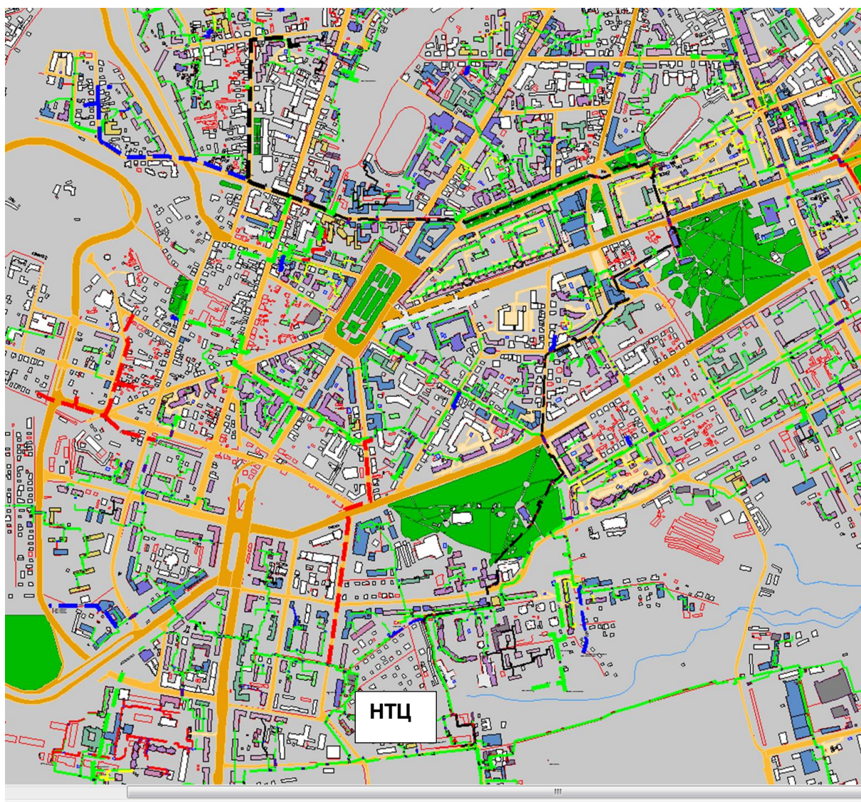
Рисунок 0.63 – Результат гидравлического расчета - расчетный путь теплоносителя от котельной НТЦ до ПТ-ПП-2.161-2017
