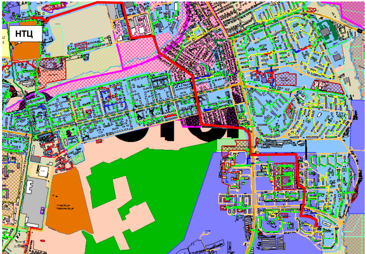
Рисунок 0.59 – Результат гидравлического расчета - расчетный путь теплоносителя от котельной НТЦ до ПТ-Малин,2 пристрой
