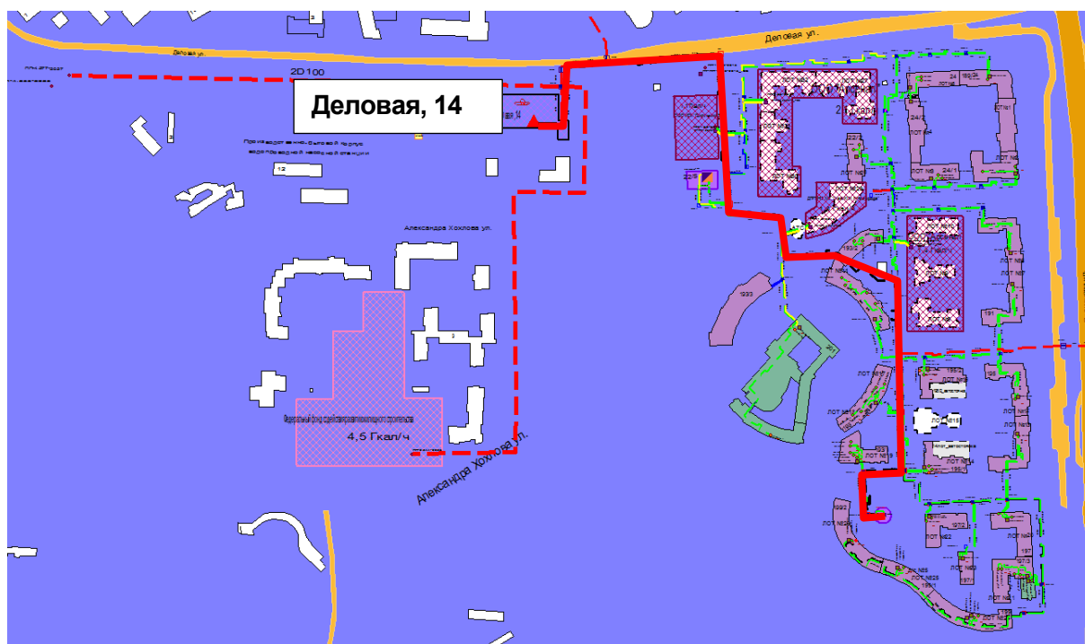
Рисунок 0.99 – Результат гидравлического расчета - расчетный путь теплоносителя от котельной Деловая, 14 до ПТ-Род.199/2_н
