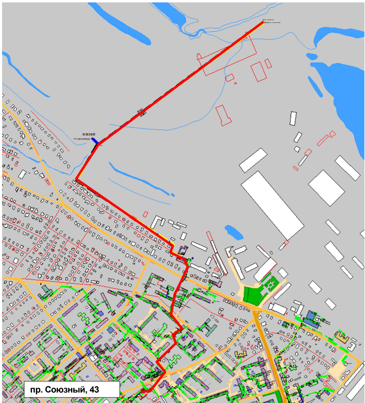
Рисунок 0.129 – Результат гидравлического расчета - расчетный путь теплоносителя от котельной пр. Союзный, 43 до ПТ-ПП-4.101/1.182-2018/2027
