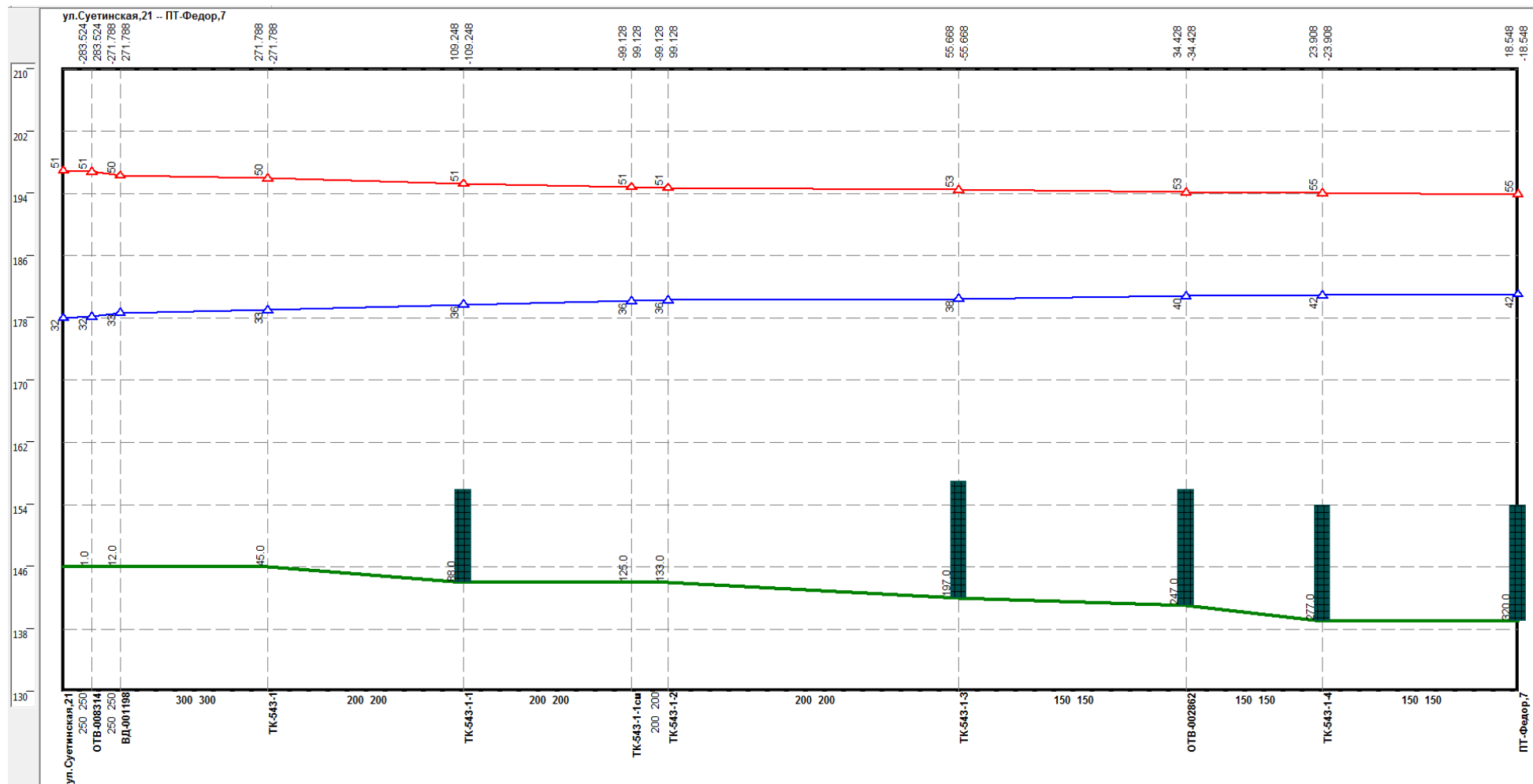
Рисунок 0.12 –Результат гидравлического расчета - график гидравлических режимов по пути теплоносителя от котельной Суетинская, 21 до ПТ-Федор, 7
