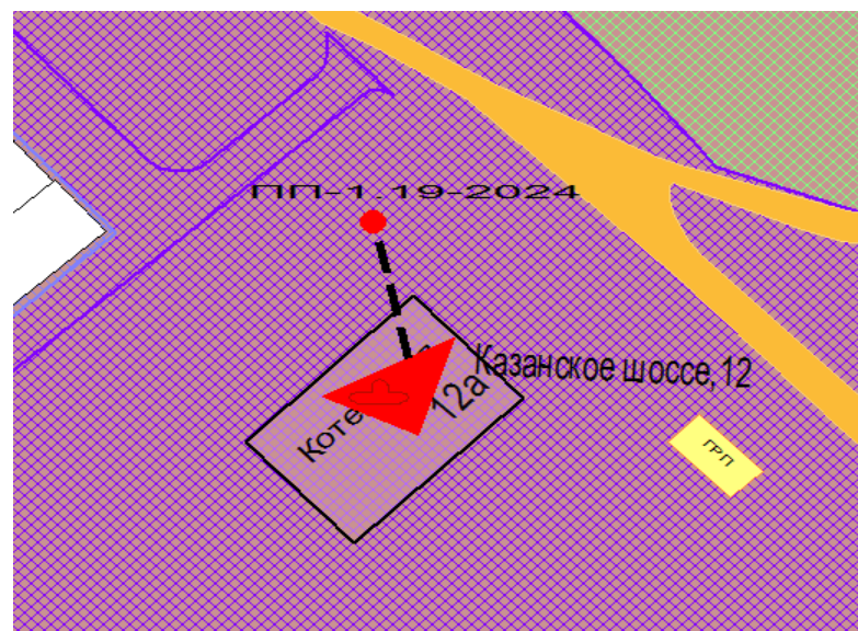
Рисунок 0.35 – Результат гидравлического расчета - расчетный путь теплоносителя от Кот. ГУ ВПО «НГТУ» до ПТ-ПП-1.19-2024
