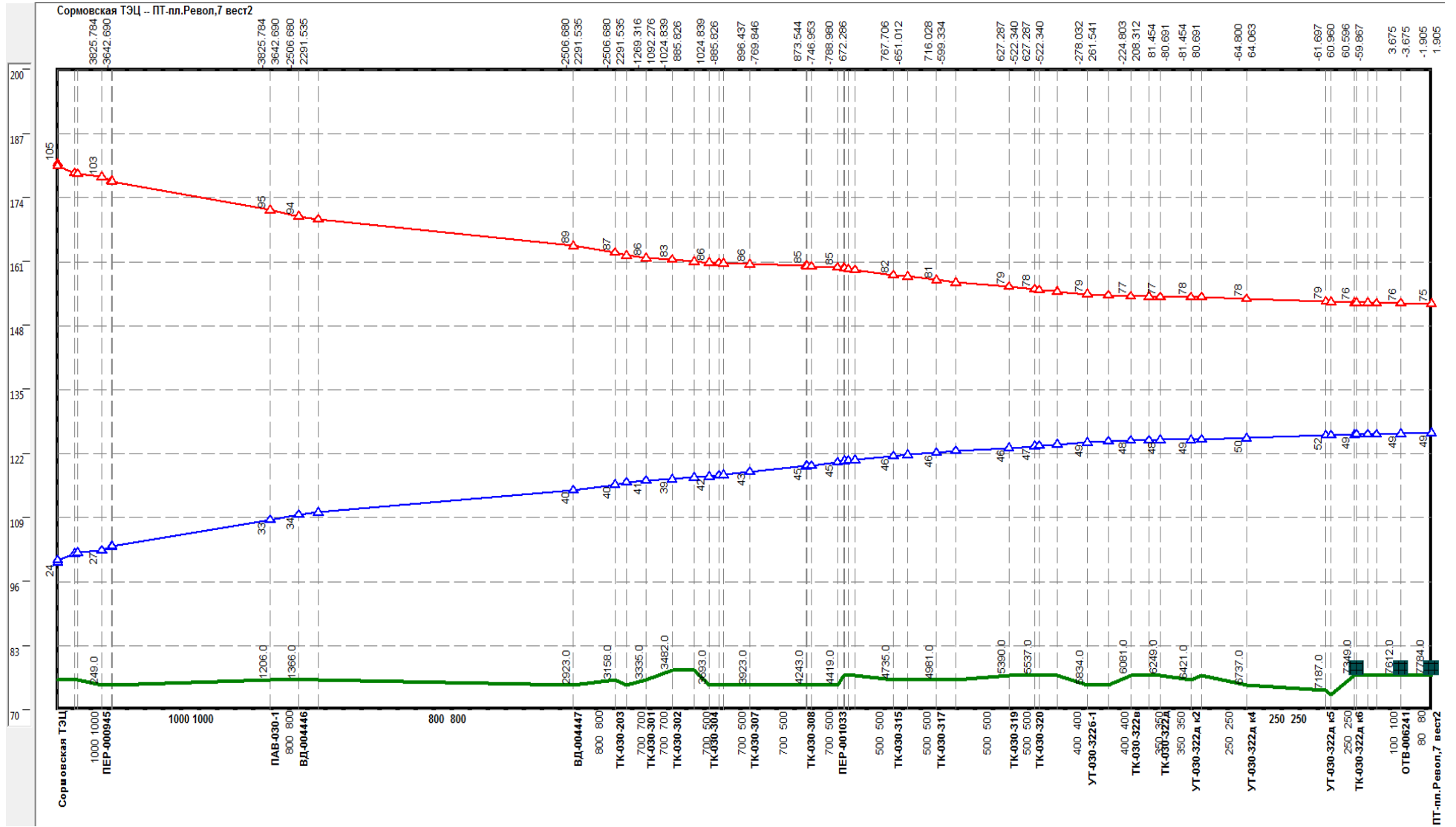
Рисунок 0.6 –Результат гидравлического расчета - график гидравлических режимов по пути теплоносителя от СТЭЦ до ПТ-пл.Револ,7 вест2.
