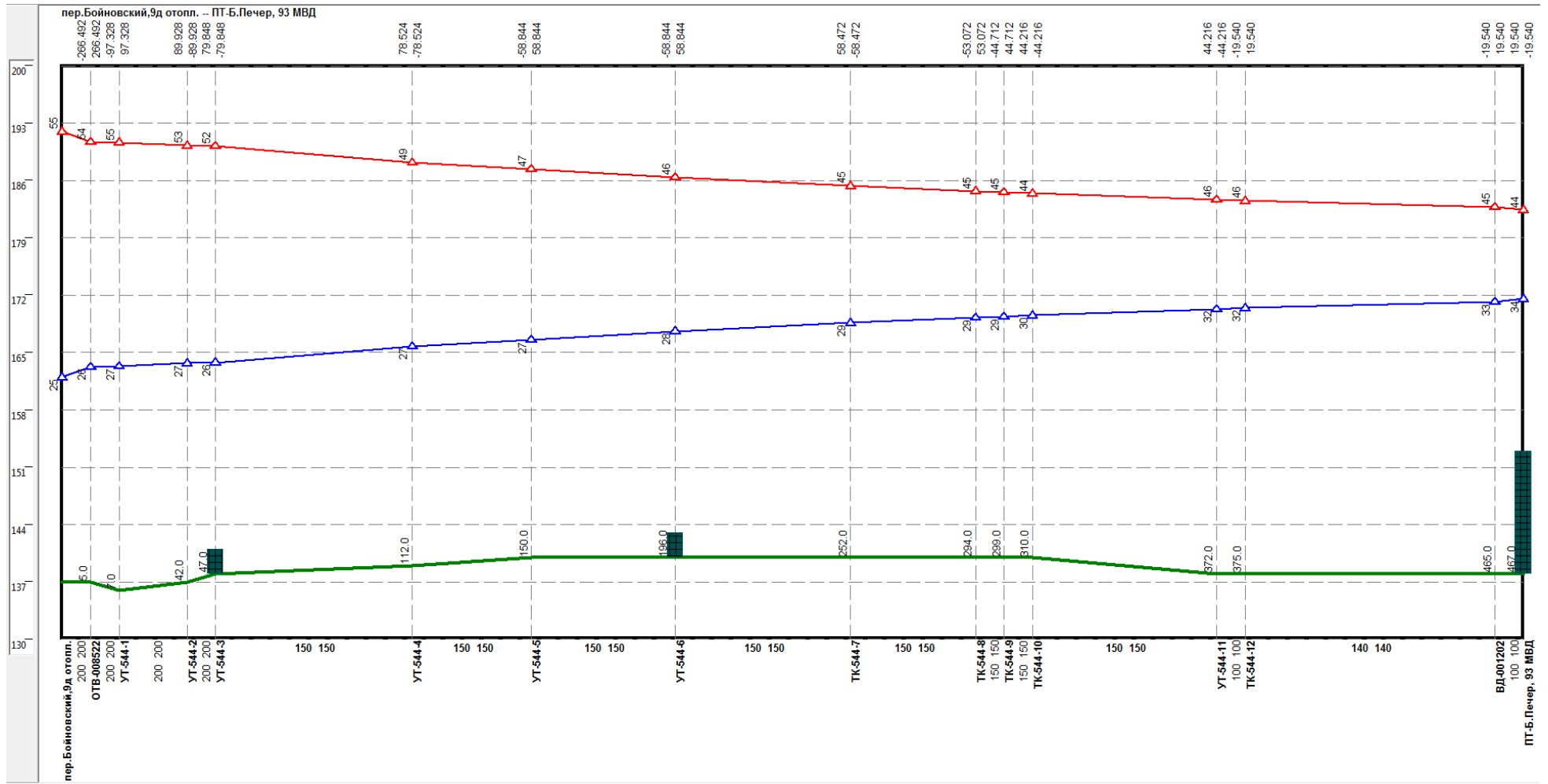
Рисунок 0.24 –Результат гидравлического расчета - график гидравлических режимов по пути теплоносителя от Бойновский, 9д до ПТ-Б.Печер, 93 МВД
