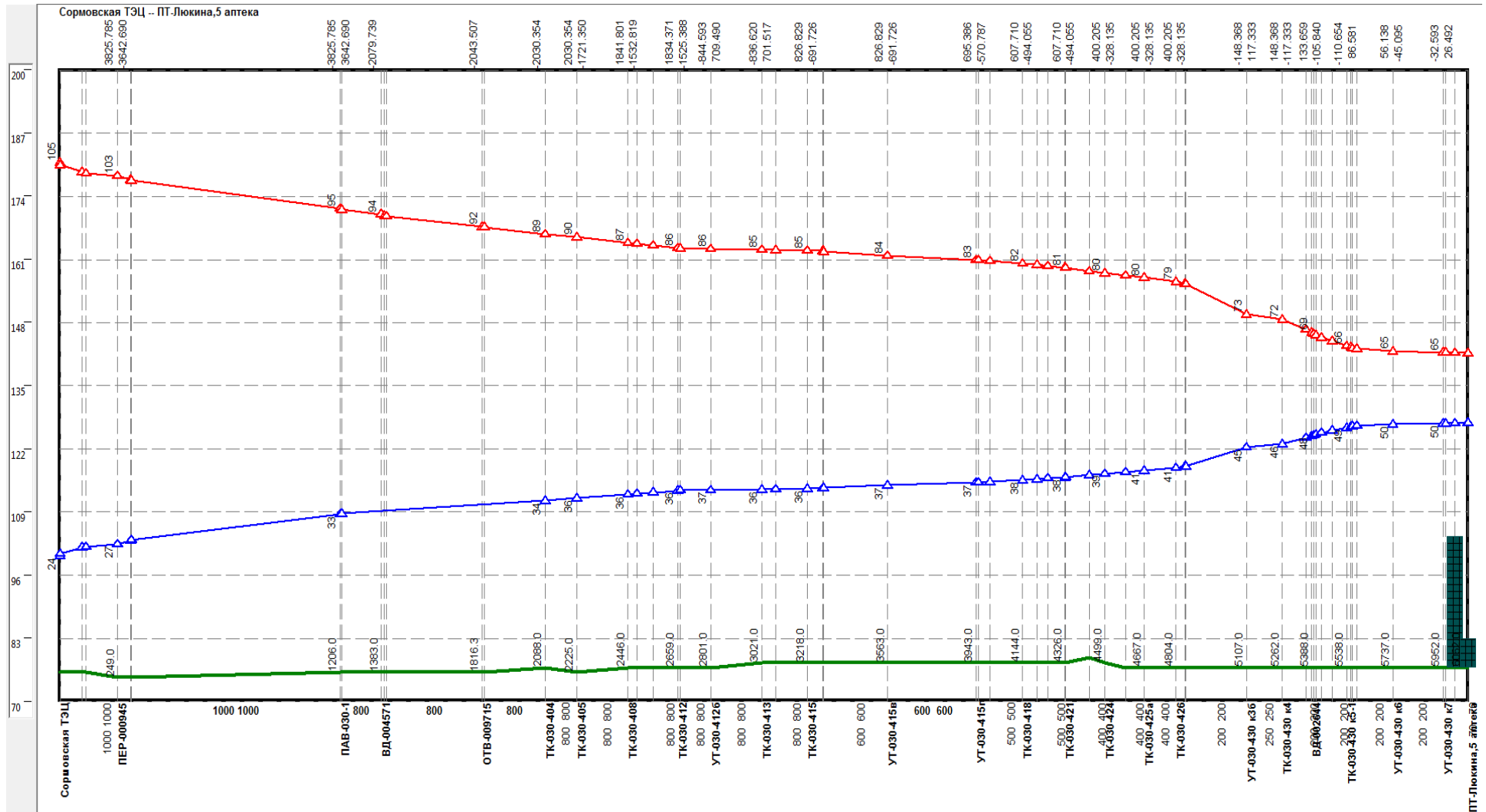
Рисунок 0.2 –Результат гидравлического расчета - график гидравлических режимов по пути теплоносителя от СТЭЦ до ПТ-Люкина,5 аптека
