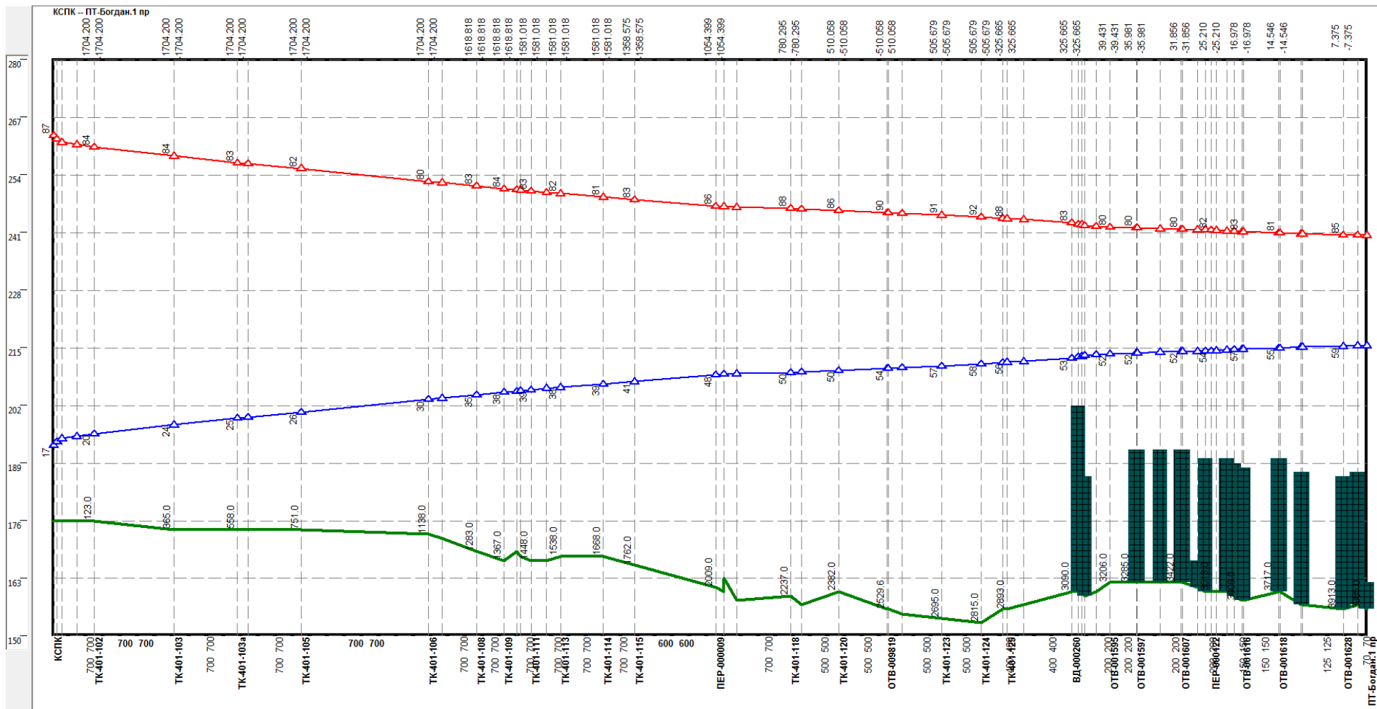
Рисунок 0.136 Результат гидравлического расчета - график гидравлических режимов по пути теплоносителя от котельной ул. Родионова, 1946 до ПТ-Богдан.1 пр
