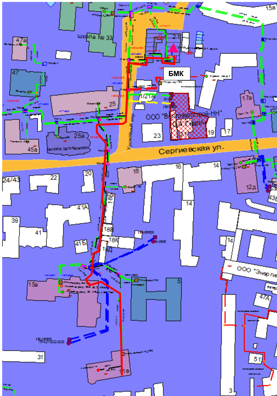
Рисунок 0.91 – Результат гидравлического расчета - расчетный путь теплоносителя от котельной Суевинская, 21 до ПТ-Нижнегород, 11в
