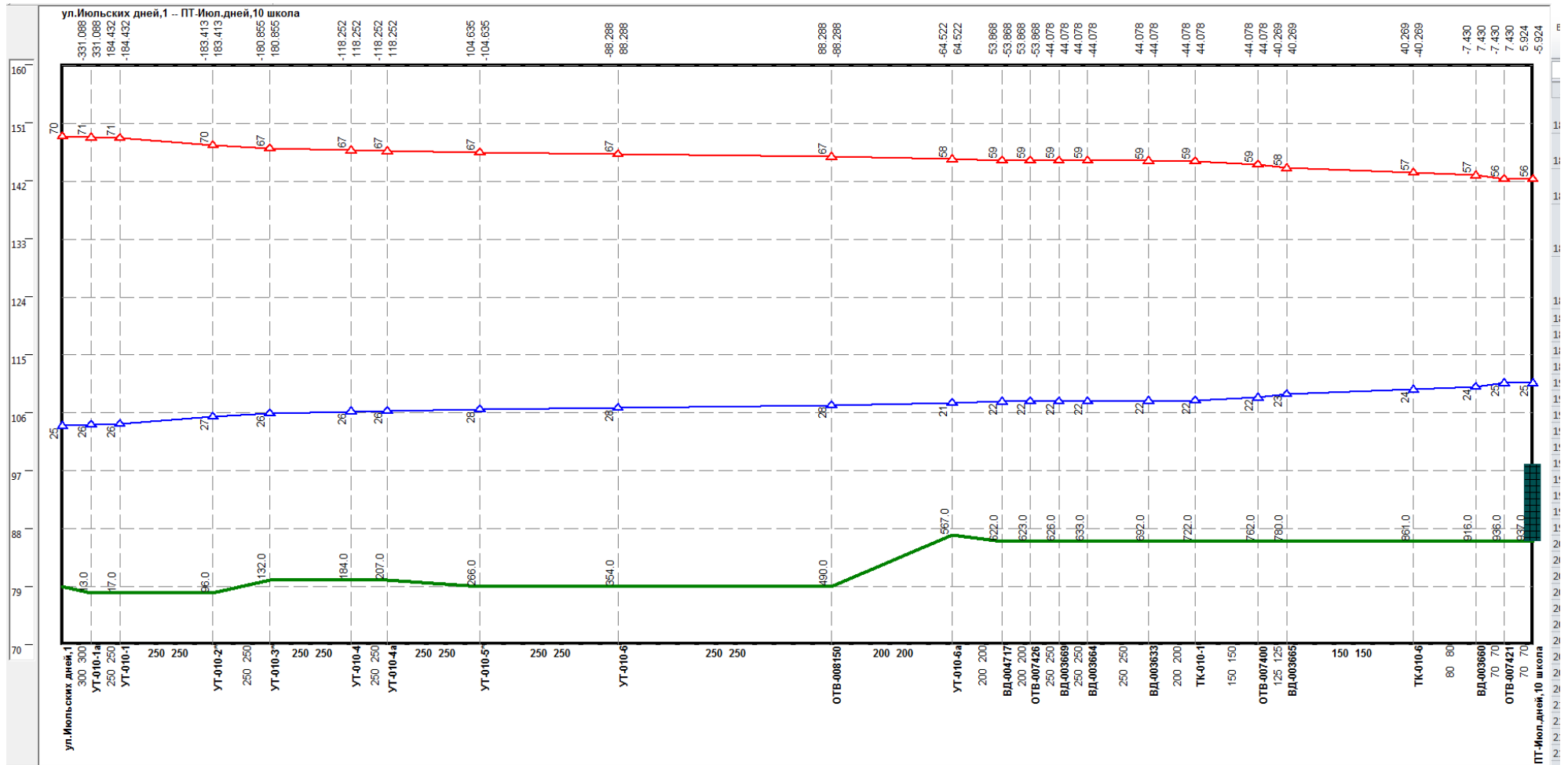
Рисунок 0.104 –Результат гидравлического расчета - график гидравлических режимов по пути теплоносителя от Июльских дней, 1 до ПТ-Июль.дней, 10 школа
