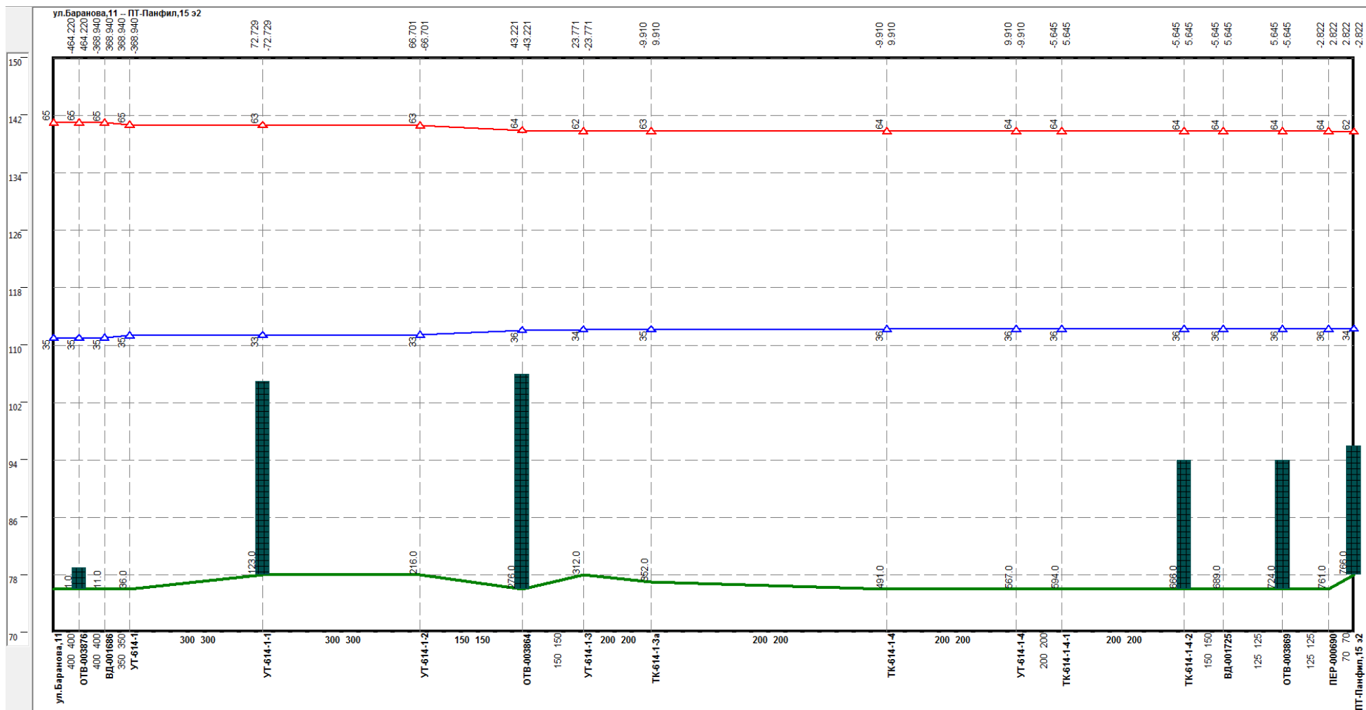
Рисунок 0.110 –Результат гидравлического расчета - график гидравлических режимов по пути теплоносителя от котельной Баранова, 11 до ПТ-Панфил,15 э2
