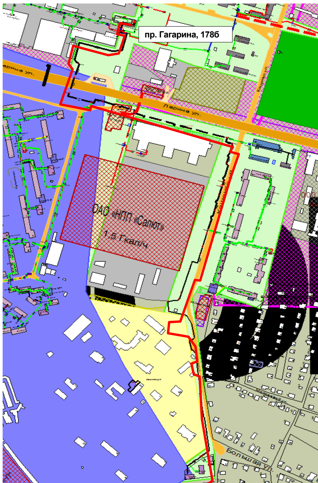
Рисунок 0.121 – Результат гидравлического расчета - расчетный путь теплоносителя от котельной пр. Гагарина, 1786 до ПТ-Кашенко, 4а
