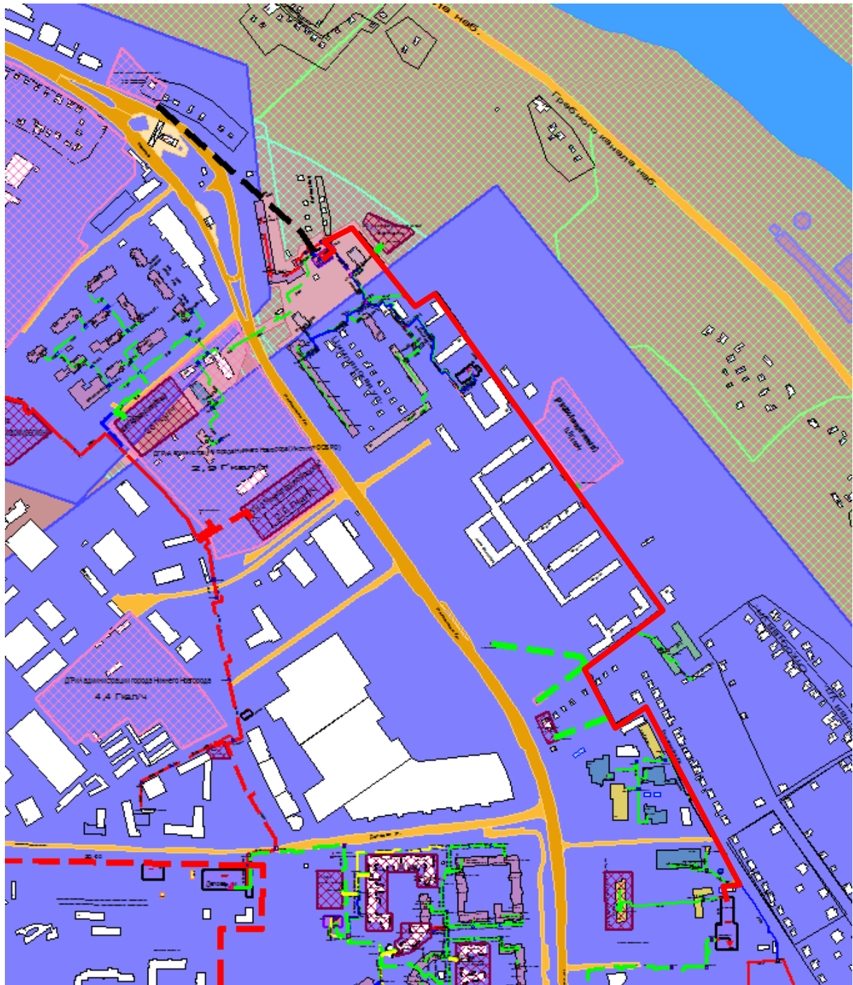
Рисунок 0.133 – Результат гидравлического расчета - расчетный путь теплоносителя от котельной ул. Родионова, 1946 до ПТ-ПП-2.67-2017
