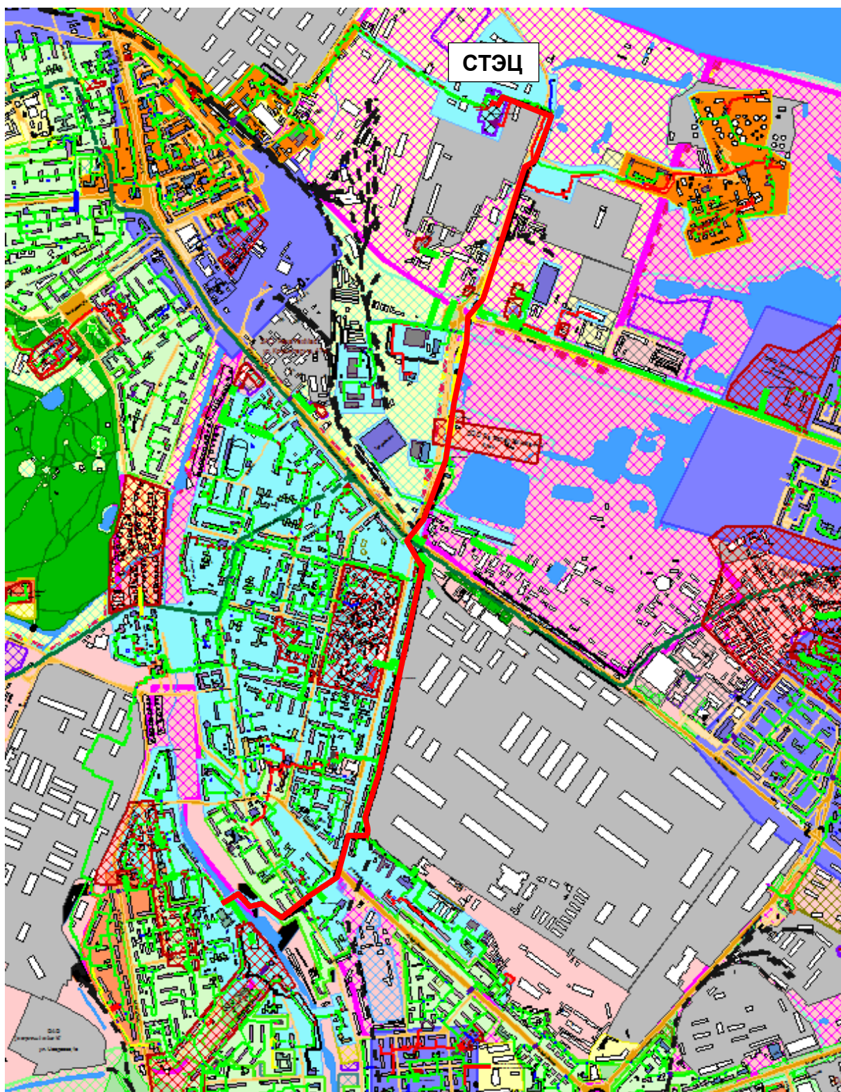
Рисунок 0.1 - Результат гидравлического расчета - расчетный путь теплоносителя от СТЭЦ до ПТ-Люкина, 5 аптека
