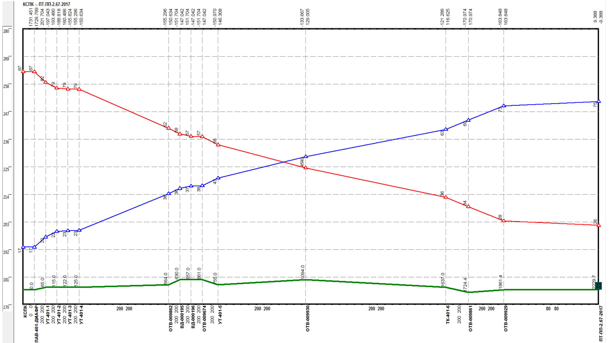
Рисунок 0.78 –Результат гидравлического расчета - график гидравлических режимов по пути теплоносителя от котельной ул. Родионова, 1946 до ПТ-ПП-2.67-2017
