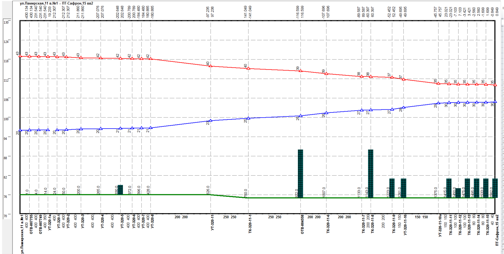
Рисунок 0.14 –Результат гидравлического расчета - график гидравлических режимов по пути теплоносителя от котельной Памирская, 11 до ПТ-Сафрон,15 вв2
