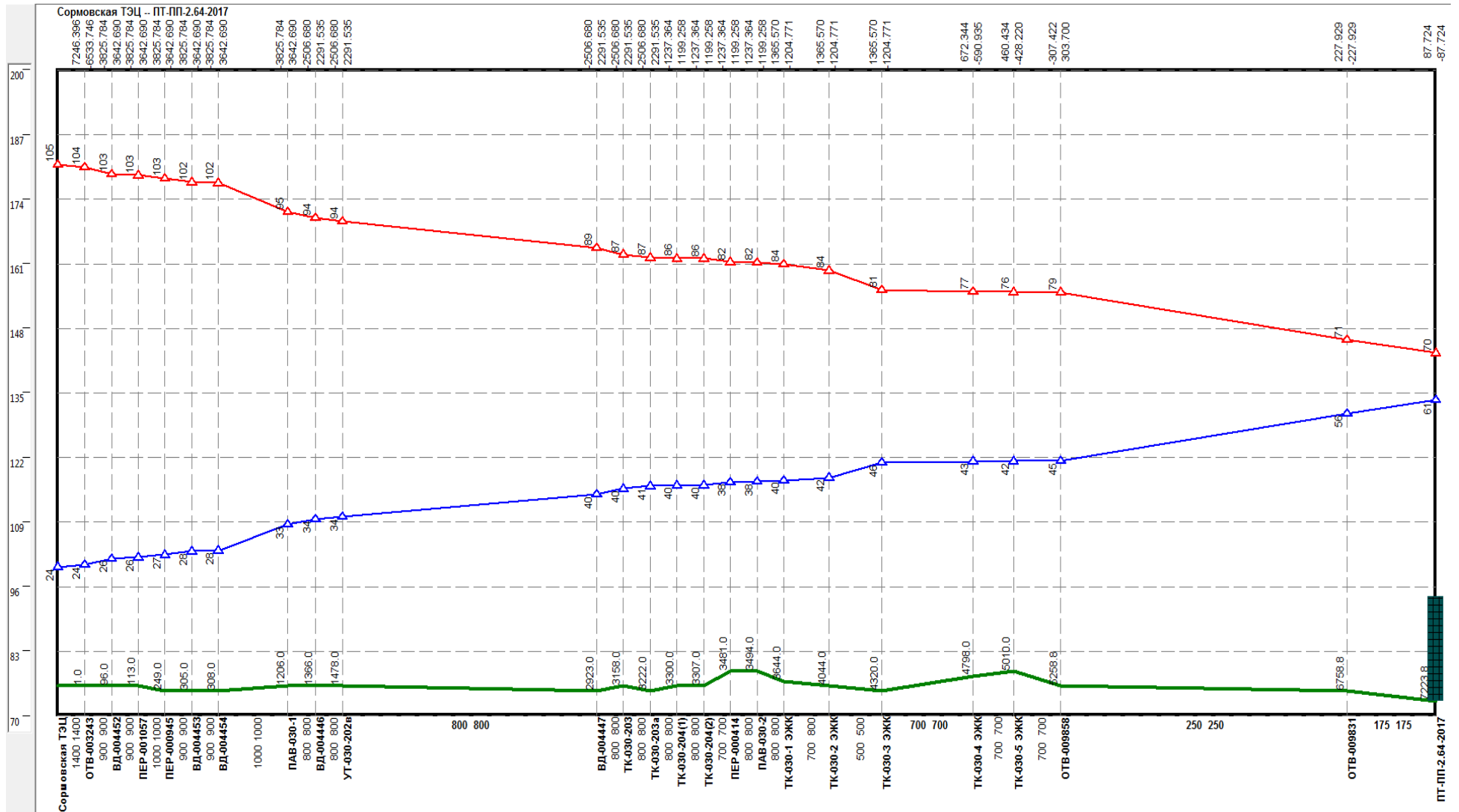
Рисунок 0.4 –Результат гидравлического расчета - график гидравлических режимов по пути теплоносителя от СТЭЦ до ПТ-ПП-2.64-2017
