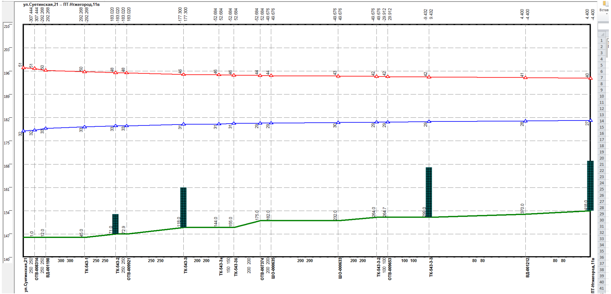
Рисунок 0.92 –Результат гидравлического расчета - график гидравлических режимов по пути теплоносителя от котельной Суетинская, 21 до ПТ-Нтжегород,11в
