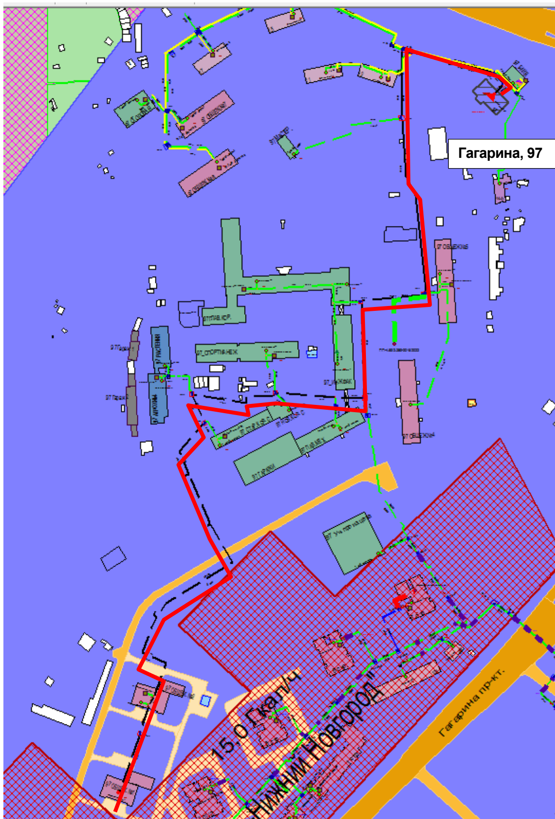
Рисунок 0.37 – Результат гидравлического расчета - расчетный путь теплоносителя от котельной пр. Гагарина, 97 до ПТ-Гагар,97 общ.№1
