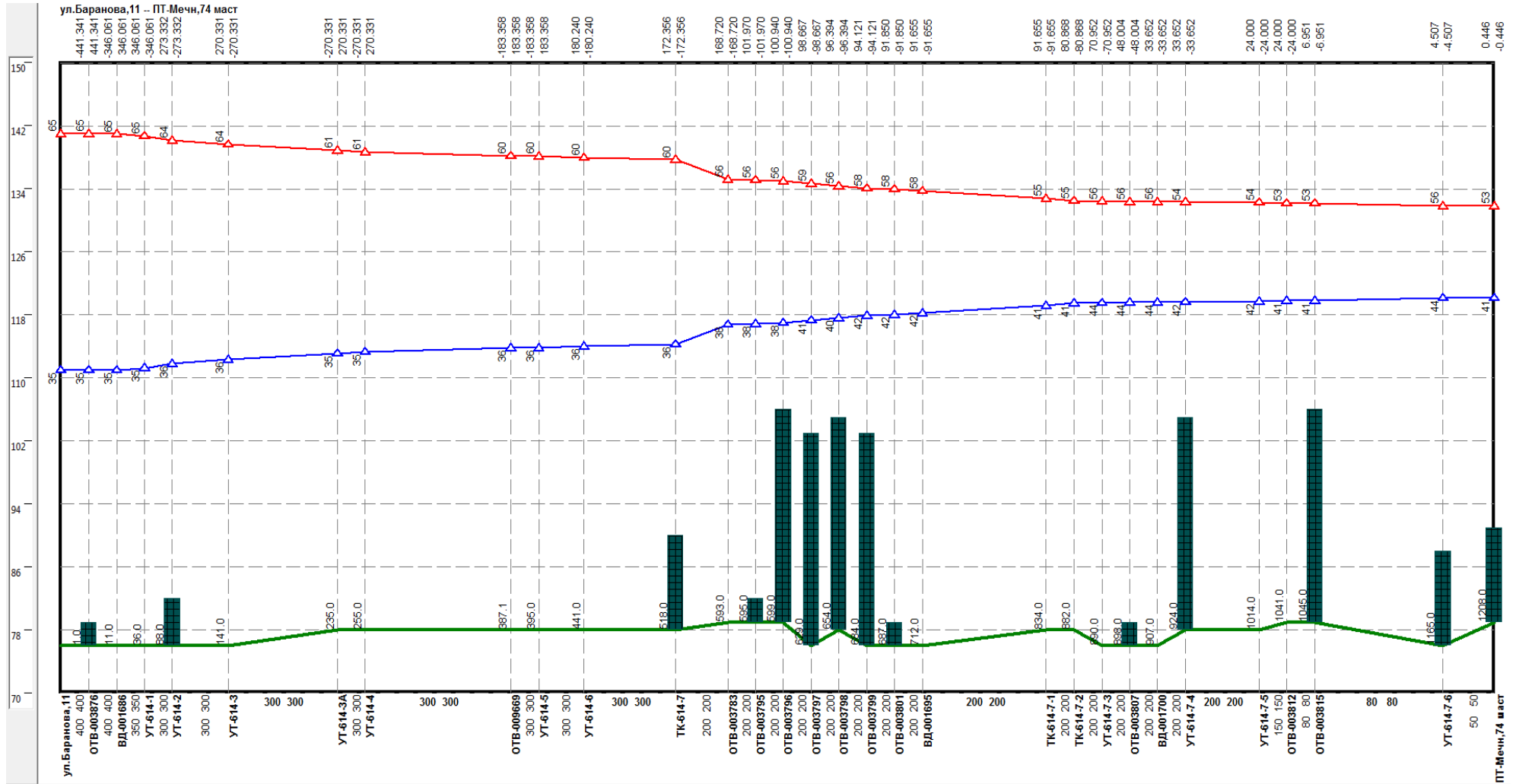
Рисунок 0.40 –Результат гидравлического расчета - график гидравлических режимов по пути теплоносителя от котельной Баранова, 11 до ПТ-Мечн,74 маст
