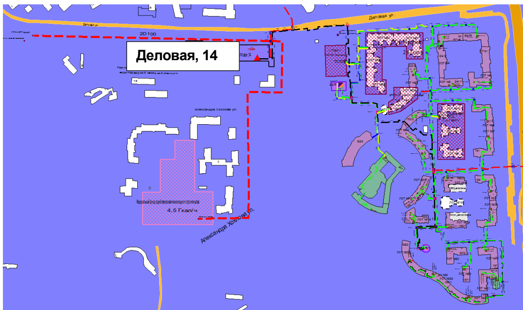
Рисунок 0.27 – Результат гидравлического расчета - расчетный путь теплоносителя от котельной Деловая, 14 до ПТ-Род.199/2_н
