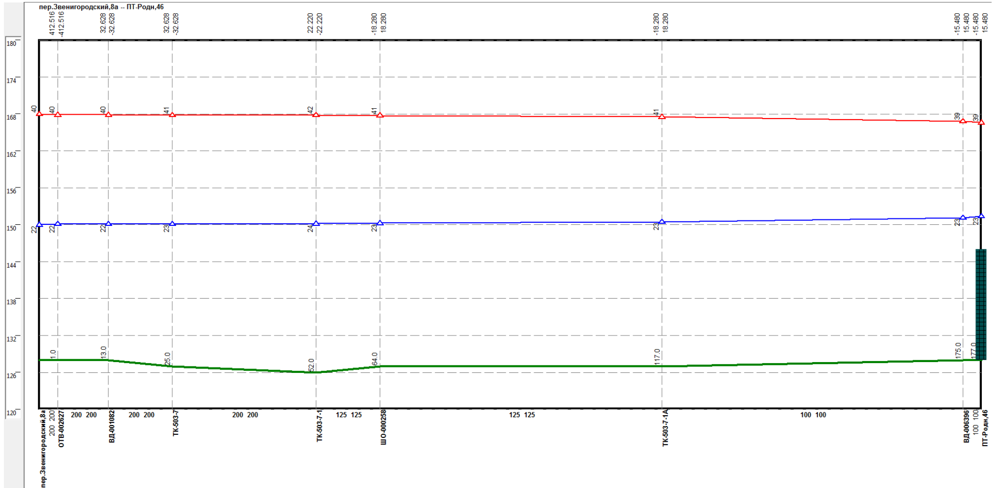
Рисунок 0.54 –Результат гидравлического расчета - график гидравлических режимов по пути теплоносителя от котельной пер. Звенигородский до ПТ-Родн,46
