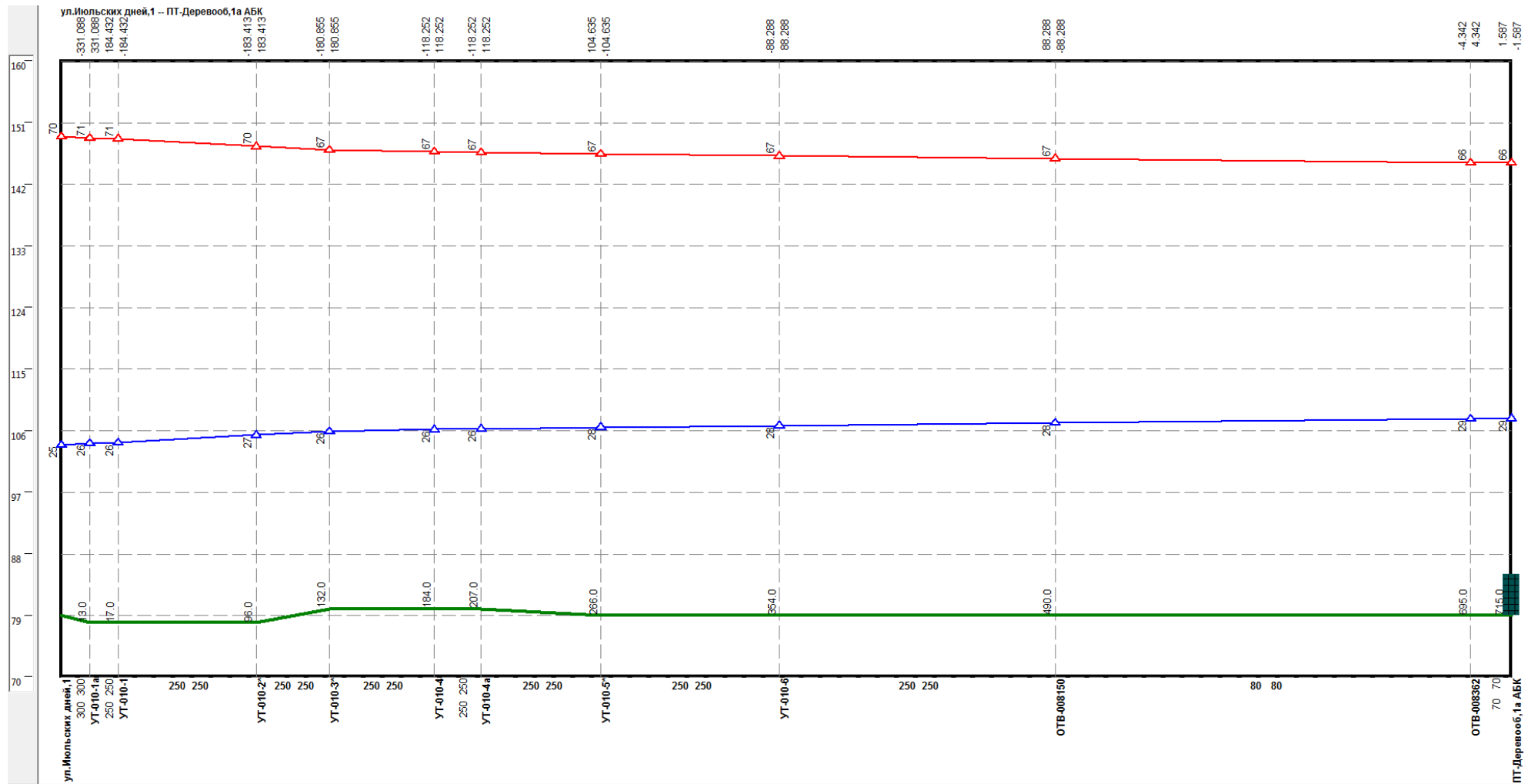
Рисунок 0.106 –Результат гидравлического расчета - график гидравлических режимов по пути теплоносителя от котельной Июльских дней, 1 до ПТ-Деревооб,1а АБК
