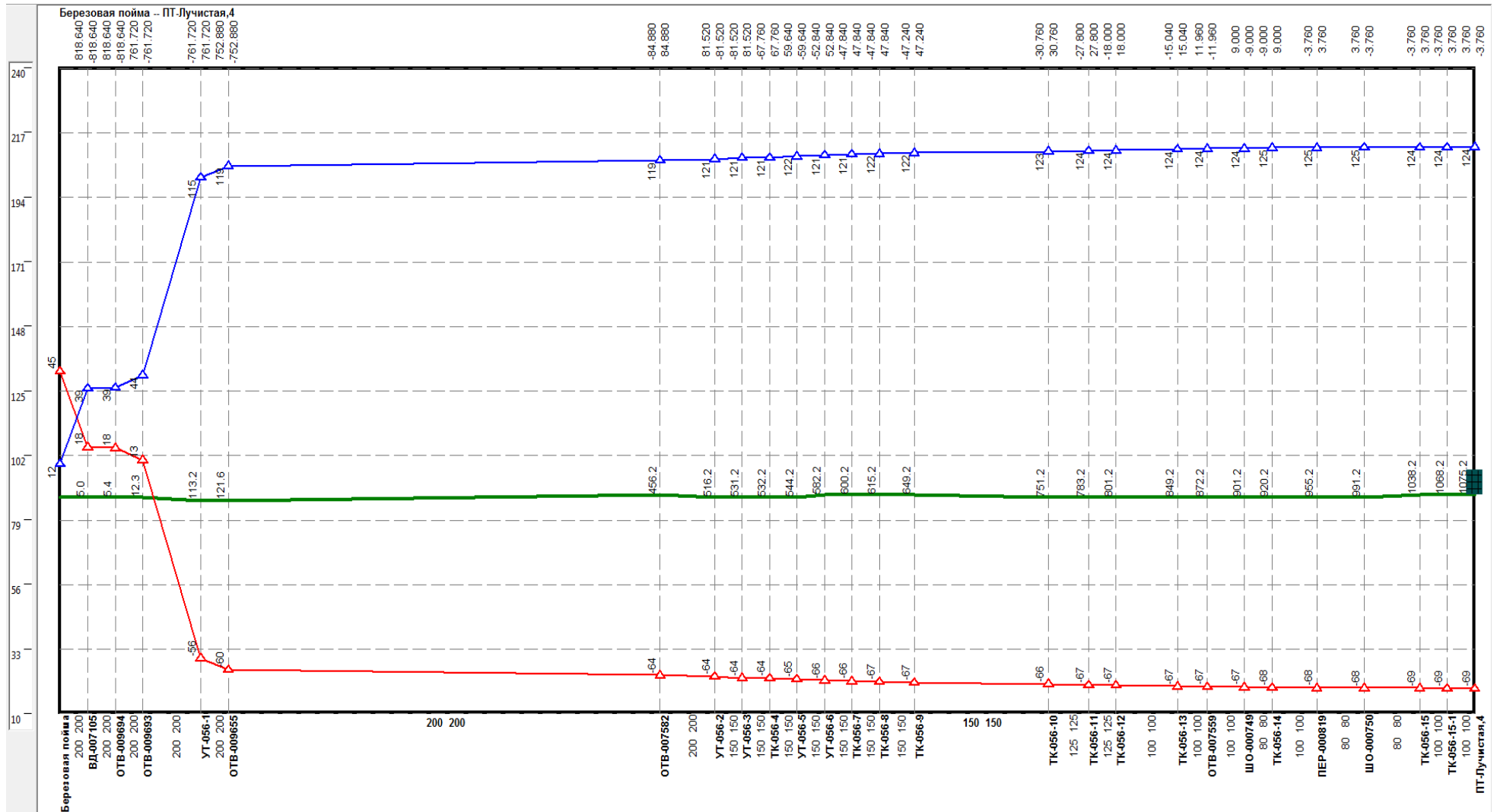
Рисунок 0.26 –Результат гидравлического расчета - график гидравлических режимов по пути теплоносителя от котельной Березовая пойма до ПТ-Лучистая, 4
