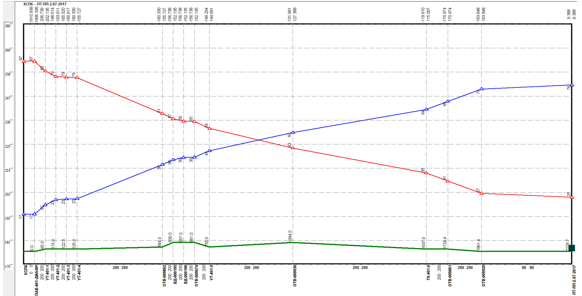
Рисунок 0.134 –Результат гидравлического расчета - график гидравлических режимов по пути теплоносителя от котельной ул. Родионова, 1946 до ПТ-ПП-2.67-2017
