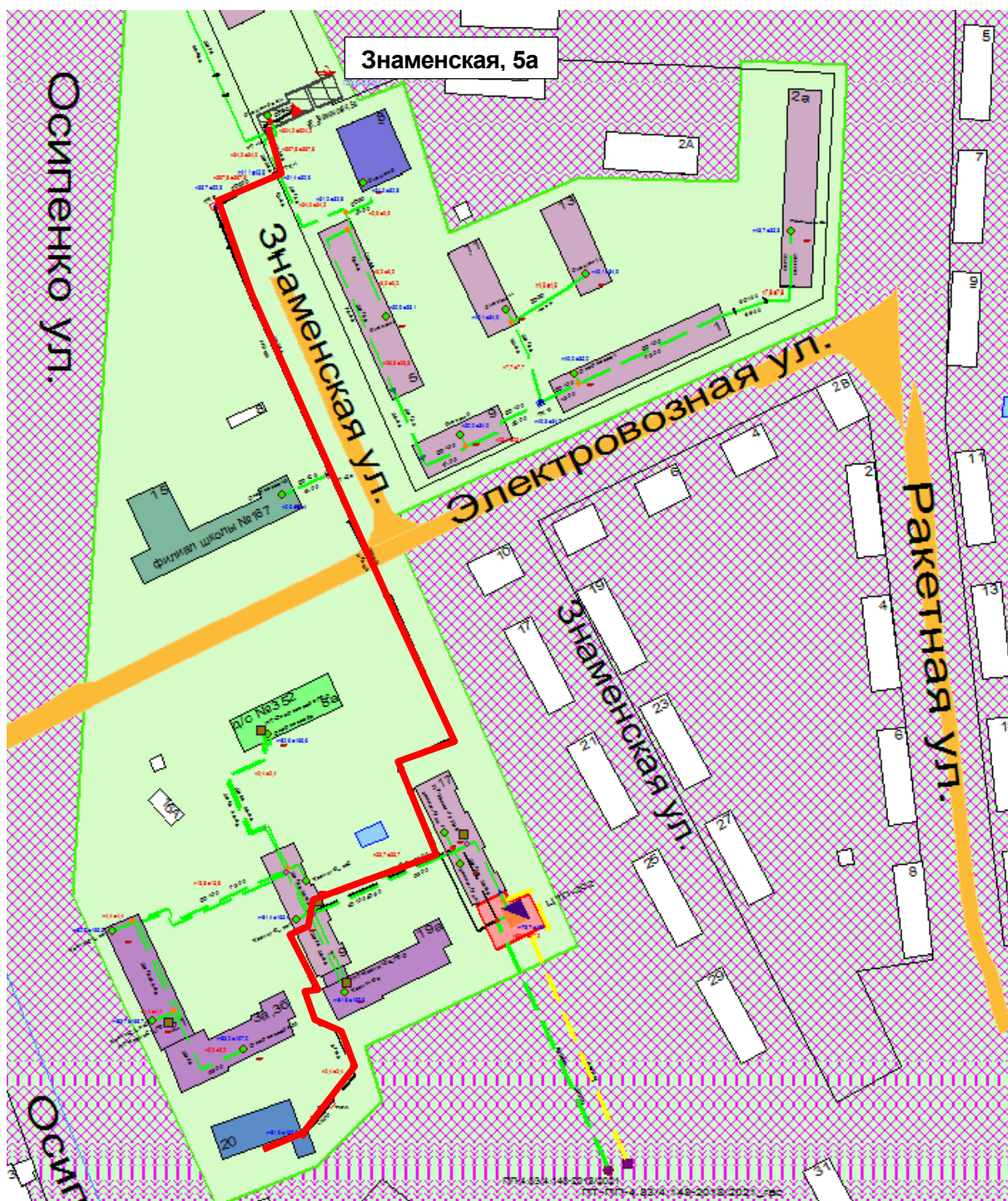
Рисунок 0.21 – Результат гидравлического расчета - расчетный путь теплоносителя от Знаменская, 5а до ПТ-Осипенко,20
