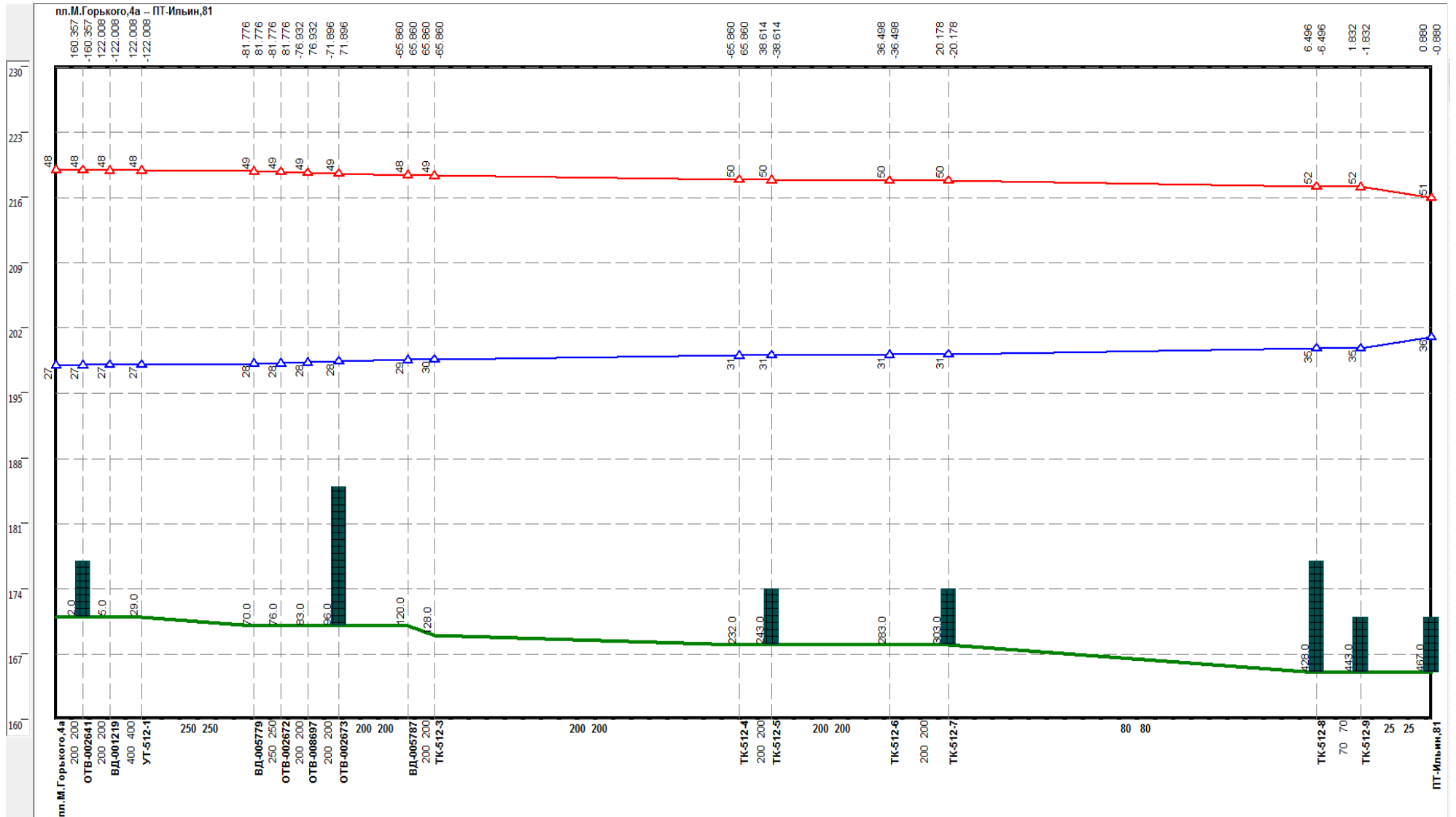
Рисунок 0.72 –Результат гидравлического расчета - график гидравлических режимов по пути теплоносителя от котельной пл. Горького, 4а до ПТ-Ильин,81
