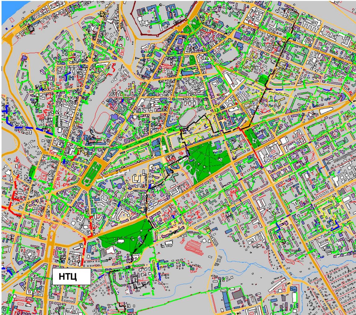
Рисунок 0.61 – Результат гидравлического расчета - расчетный путь теплоносителя от котельной НТЦ до ПТ- ПП-2-50-2015.
