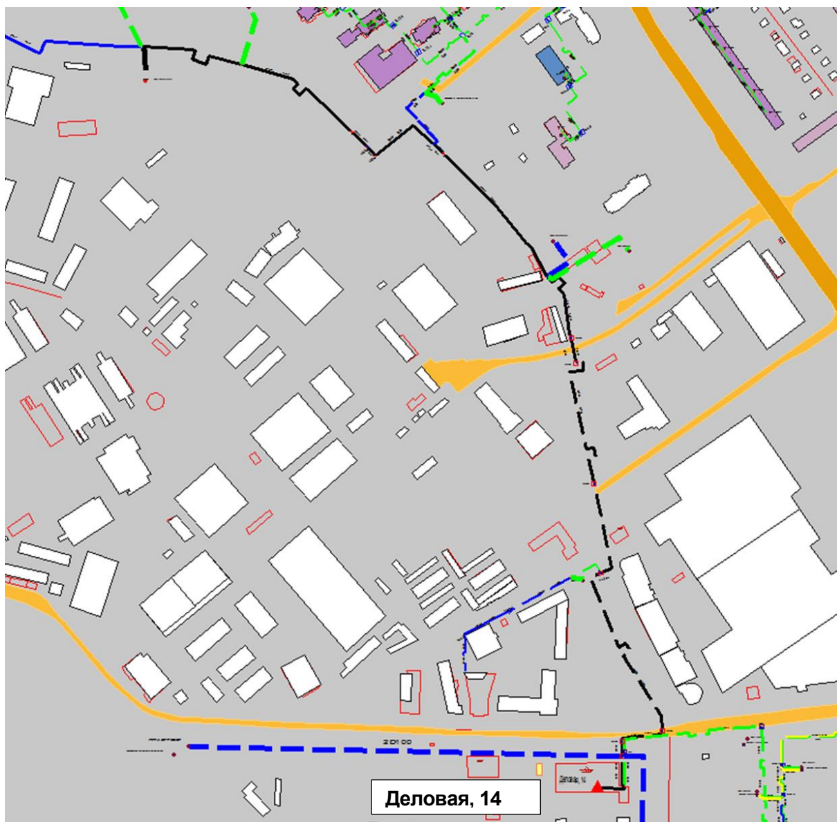
Рисунок 0.29 – Результат гидравлического расчета - расчетный путь теплоносителя от котельной Деловая, 14 до ПТ-ПП-2.99-2017-2018
