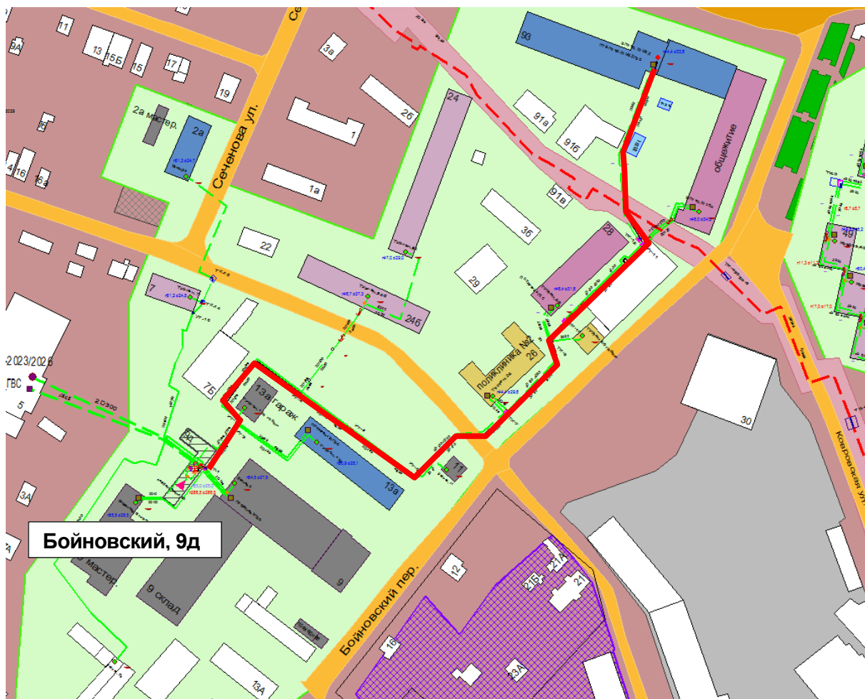
Рисунок 0.23 – Результат гидравлического расчета - расчетный путь теплоносителя от Бойновский, 9д до ПТ-Б.Печер, 93 МВт
