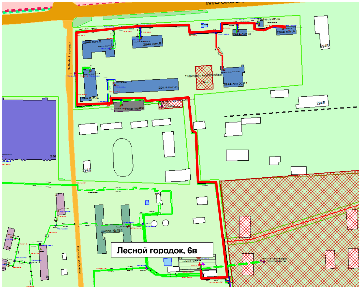
Рисунок 0.19 – Результат гидравлического расчета - расчетный путь теплоносителя от Лесной городок 6в до ПТ-Моск.ш,294в лит.А
